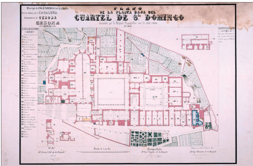
Fig. 2. Plano de la planta baja del cuartel de Santo Domingo. Archivo General Militar de Madrid. PL Signatura: GE-29/8.
