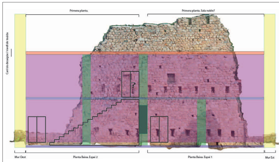
Fig. 11. Esquema arquitectònic de la torre d'en Pega. Imatge base: Lluís Prat Busquets, delineant. Diputació de Girona-Servei de Monuments.
