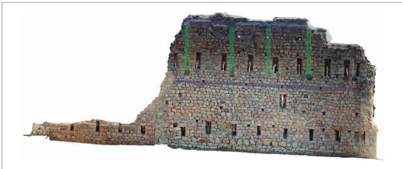
Fig. 3. Proposta de funcionament de l'entramat de passos de ronda. En color morat es marquen els possibles nivells de circulació aeris. Els trams verds assenyalen uns possibles tornapunts de sustentació. Imatge base realitzada per Lluís Prat Busquets, delineant. Diputació de Girona-Servei de Monuments.
