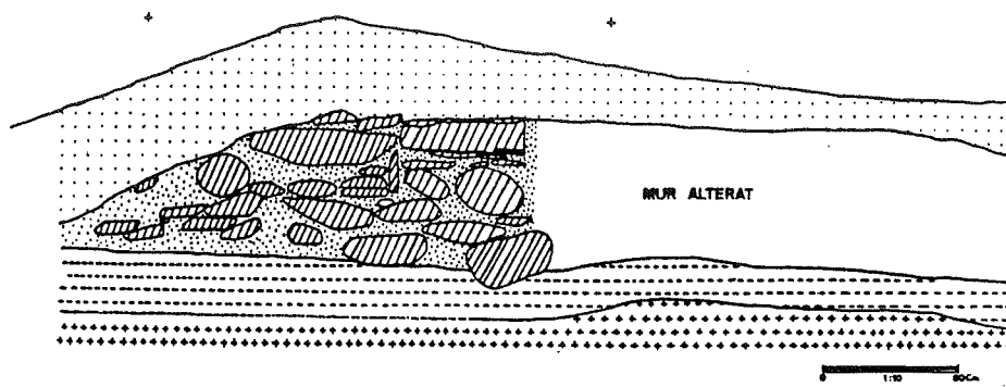
SONDEIG 'B' ALCAT NORD
