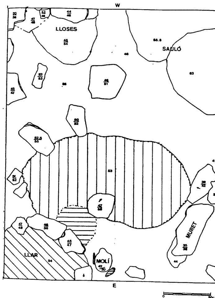
PLANTA SONDEIG 'D'
