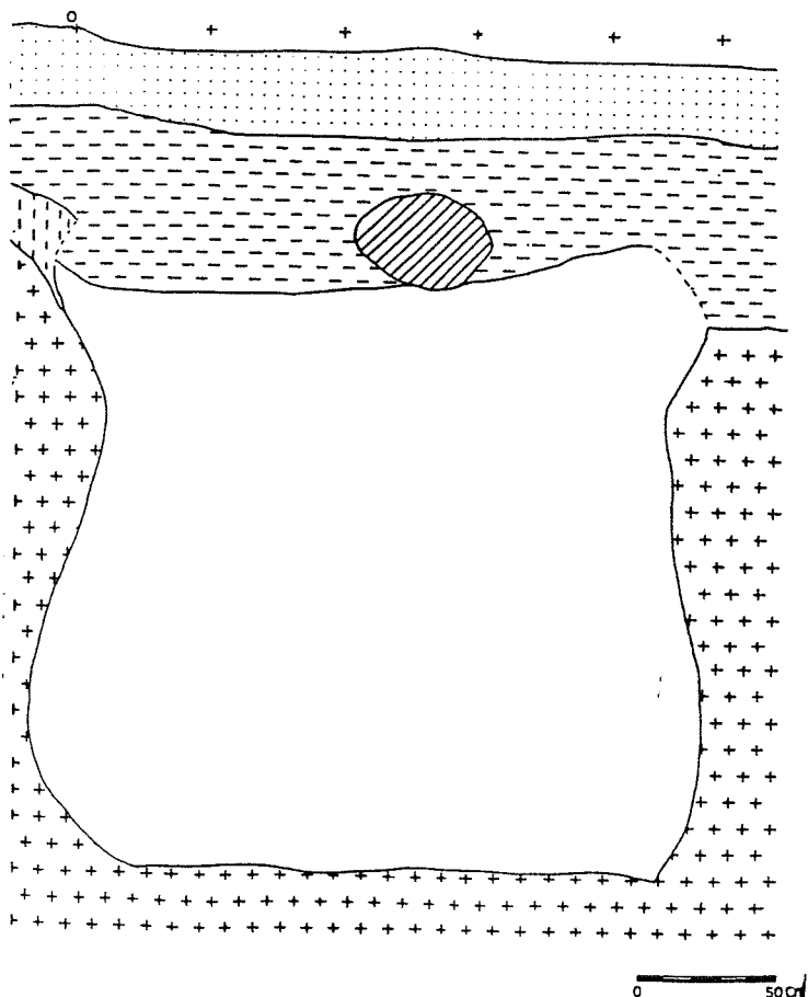
SONDEIG 'C', ALCAT NORD (SITJA)
