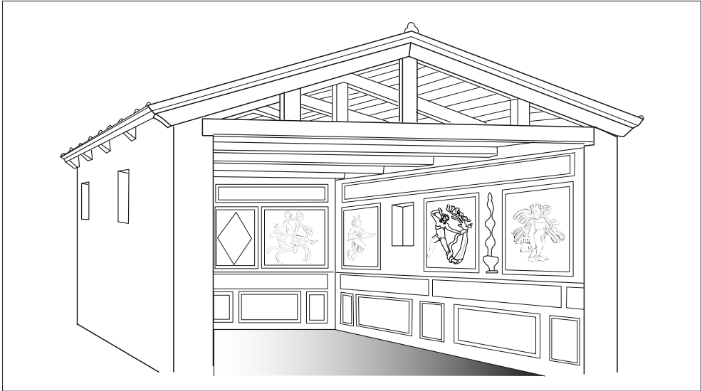
179. Estructura teòrica de l'embigat i suport de teulada en una construcció d'època romana.
