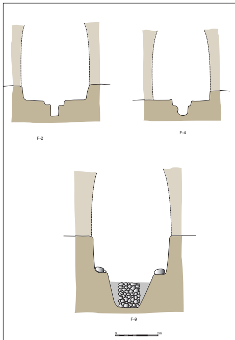
102. Collet Est. Secció i prolongació vertical de tres forns de calç.
