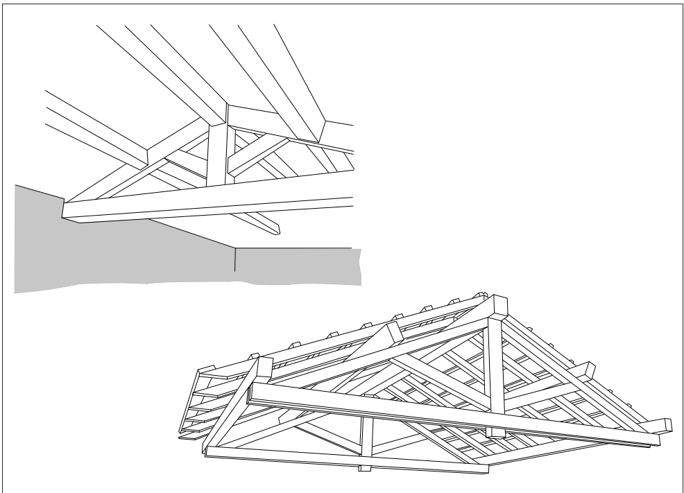
180. Diverses solucions en la construcció de l'estructura de fusta de suport d'una teulada amb mètodes tradicionals.
