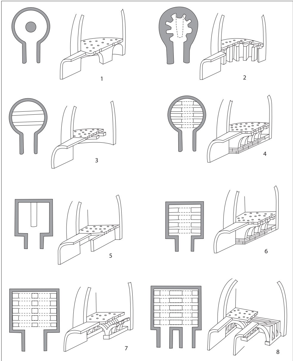
48. A) Circulars. 1: Sostingut amb pilar central; 2: Sostingut amb mur radial; 3: Amb dos arcs; 4: Amb corredor central. B: Quadrats. 5: Amb mur axial; 6: Amb corredor central; 7: Sostingut amb doble corredor; 8: Amb doble prae-furnium . Tipologia segons Cuomo di Caprio 1971-72 i 2007 ( Ceramica in Archeologia 2)
