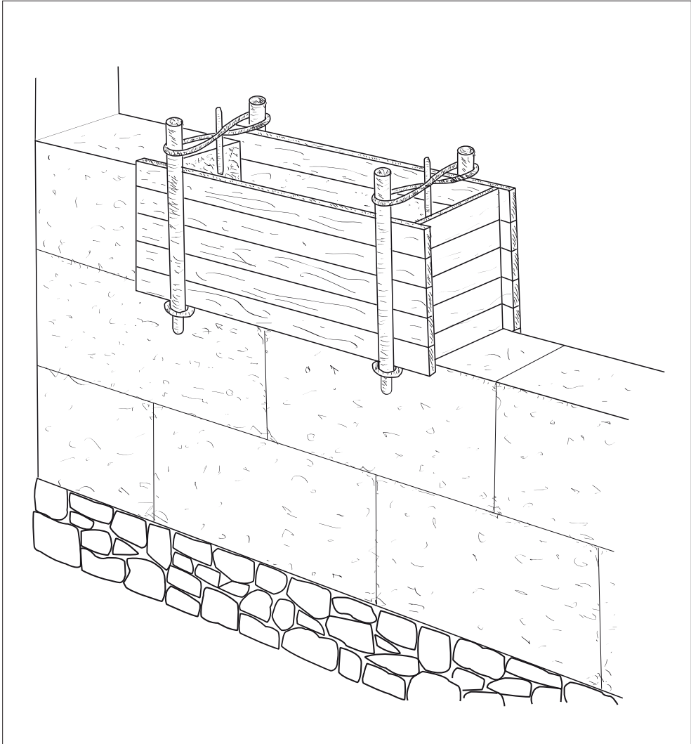
11. Esquema gràfic d'una tapiera que s'omplia amb argila mesclada amb palla i altres components i que, de vegades, s'abeurava amb calç per donar-li més consistència. En acabar un tram (tapió), calia moure l'estructura cap a un cantó o per sobre.
