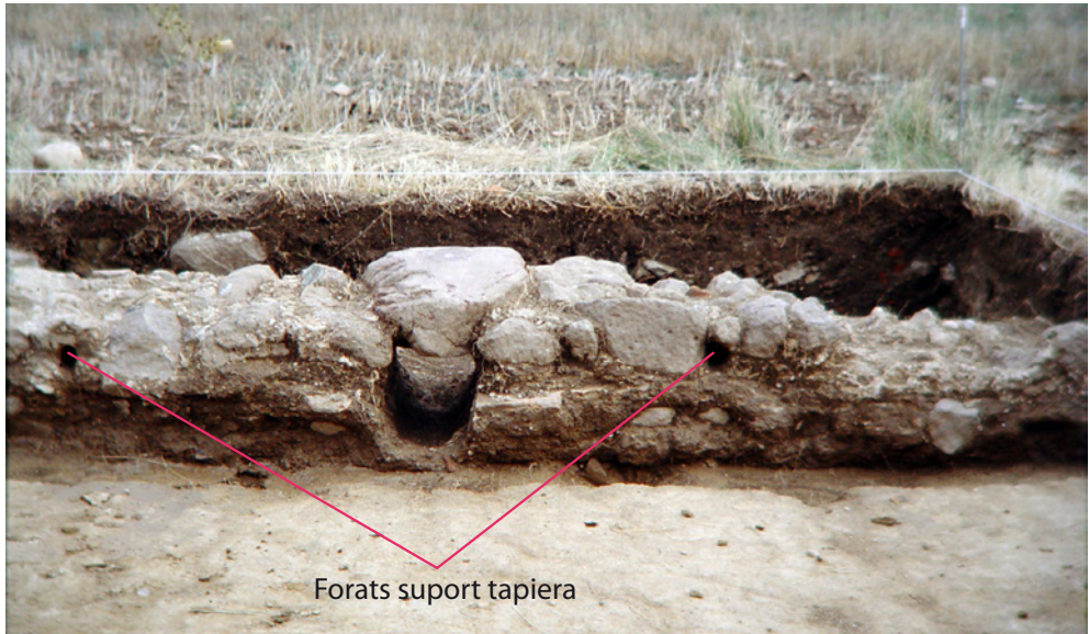
15. Puig Rodon. En la mateixa línia que l'exemple anterior, en aquest cas, podem apreciar els forats en negatiu dels posts de sosteniment de la tapiera. En acabar, aquests orificis quedaven amagats pel revestiment exterior que uniformitzava el conjunt.
