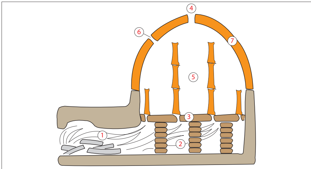
47. Esquema de les parts d'un forn: 1: praefurnium ; 2: fornax o fogaina; 3: garbell amb els espiralls; 4: tir; 5: laboratorium ; 6: speculum ; 7: volta.
