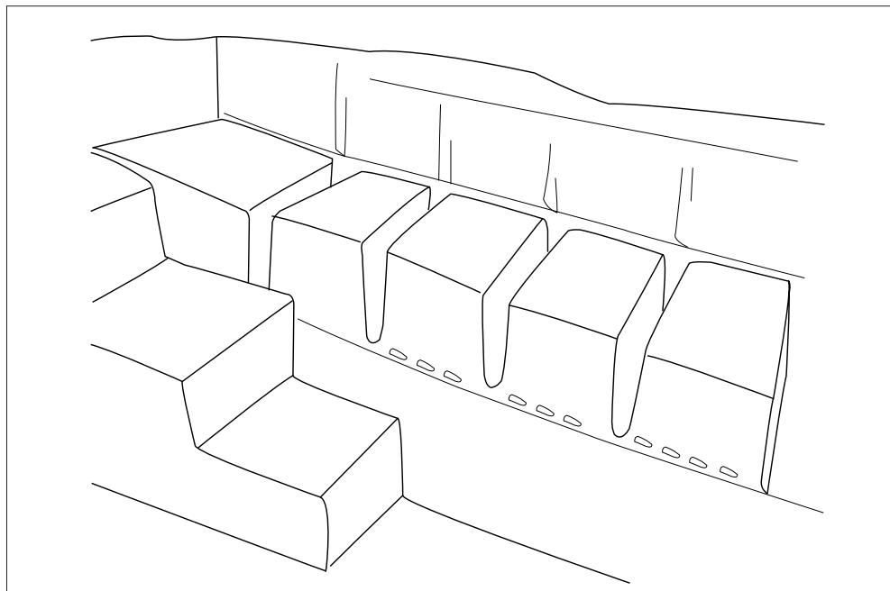
52. Esquema del procés extractiu dels blocs de pedra d'una pedrera romana
