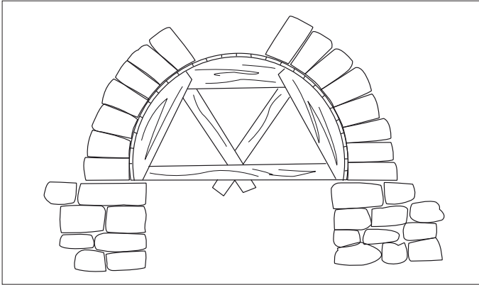
181. Exemple de cintra de fusta per bastir arcs i voltes.
