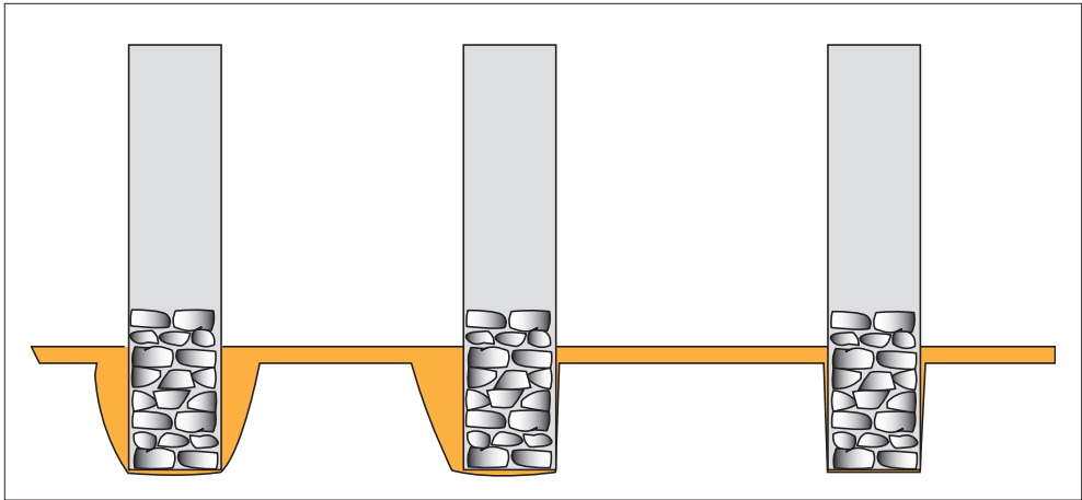
187. Esquema constructiu de la gran majoria de murs d'època romana on es poden observar els tres tipus de rasa constructiva: rasa amb reble a banda i banda, rasa amb reble només a una banda i rasa a sac, on s'ajusta la fonamentació al tall realitzat.
