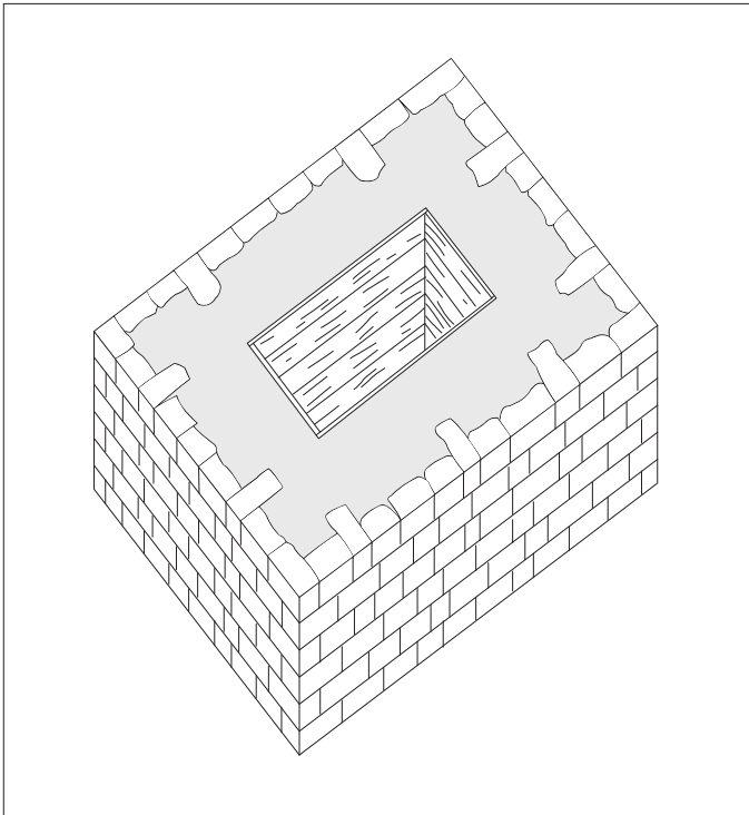
119. Aquesta imatge il·lustra la tècnica constructiva utilitzada per bastir les torres tetràriques de les muralles de Gerunda. Els carreus parallelograms de gres defineixen la cara externa ( opus quadratum ) i uns taulons de fusta la cara interna amb la voluntat de deixar un buit interior. L'espai entre els blocs i l'encofrat s'omple de pedruscall i morter de calç ( opus caementicium ). De tant en tant un dels carreus es disposava de través per assegurar una imbricació entre els dos elements. En acabar un tram, s'iniciava el següent.
