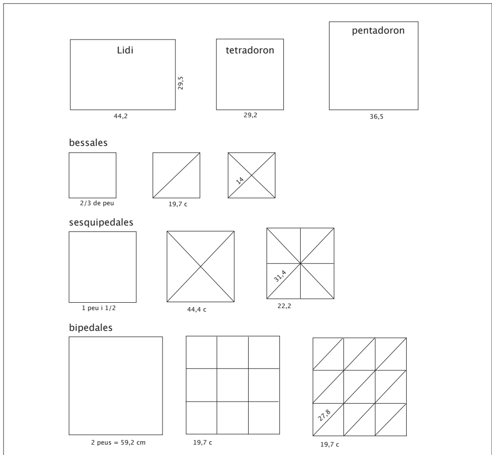
31. Esquema dels diferents mòduls de rajol documentats en època romana en base als exemples identificats en aquestes contrades.
