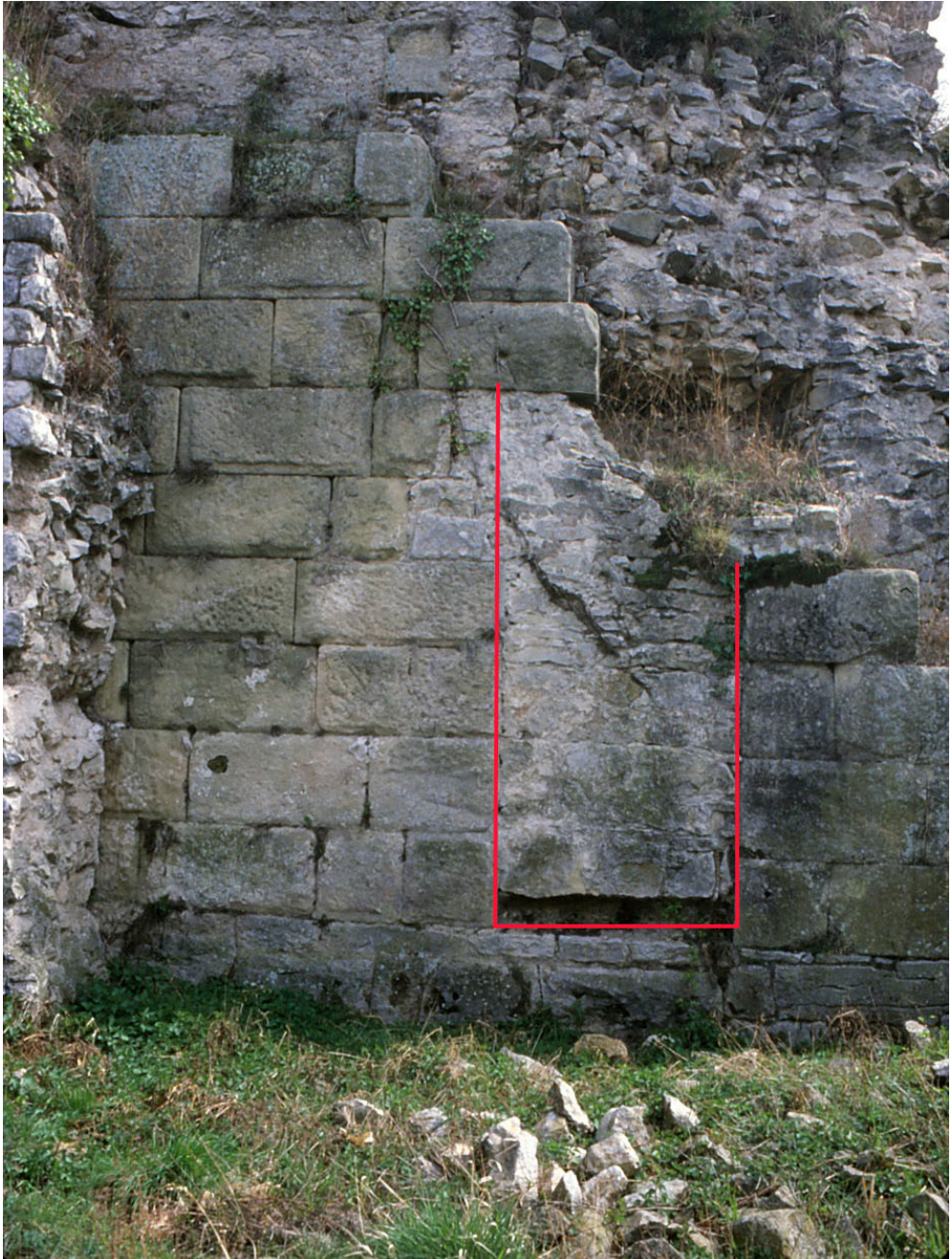
73. Girona, castell de Gironella, torre núm. 2. Exemple d' opus quadratum amb encoixinat. Fixem-nos en la porta d'accés original (època tetràrquica).
