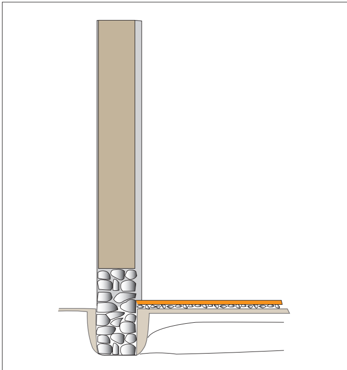
192. Esquema constructiu d'un edifici d'època romana on podem apreciar els diversos elements que s'han mencionat al llarg del llibre: una rasa de fonamentació on es basteixen els fonaments, per sobre el sòcol vist i, al damunt, la paret de tàpia. Un cop enllestit el sòl, d' opus signinum en aquest exemple, el mur es remolinava i, si convenia, es pintava.
