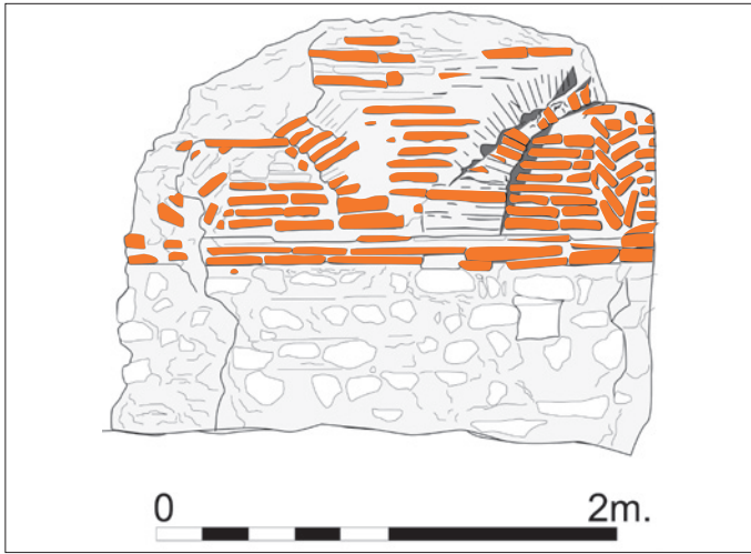
19. Torre del Fum. Monestir. Els rajols s'usaven, també, en altres tipus d'estructures. Un bon exemple és la cúpula, parcialment conservada, d'un edifici de planta octogonal de vers el 400.
