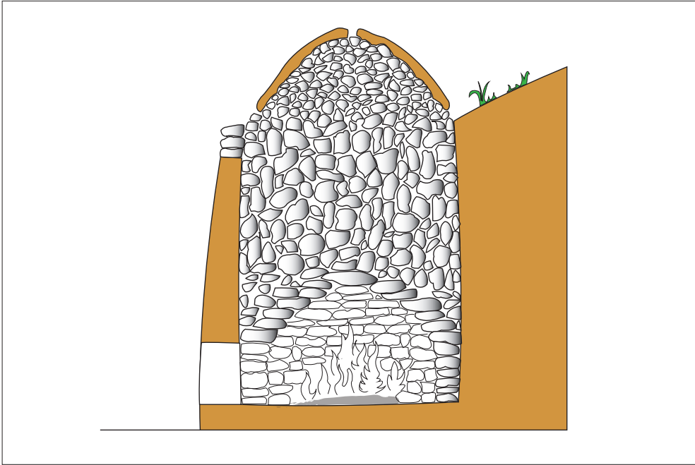
100. Reconstrucció del forn de calç descrit per Cató.
