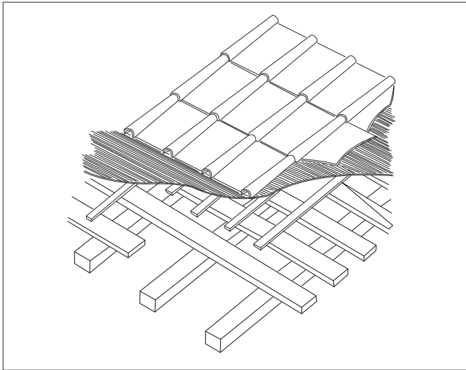
198. Esquema de funcionament d'una coberta d'un edifici romà. Per sobre les bigues s'hi documenta un entramat de palla o canyes sobre el qual es disposen posteriorment tegulae i imbrices.
