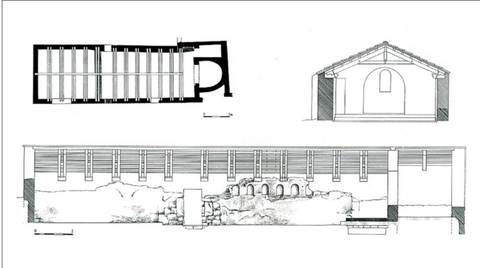
118. Empúries, Neàpolis. L'imponent mur d' opus caementicium que definia el costat de tramuntana del caldarium del balaneion hellenístic, s'ha conservat —cas únic— sencer en alçada cosa que permet observar els retalls paral·lels que permetien encaixar-hi les bigues del sostre que cobria la cella memoriae .
