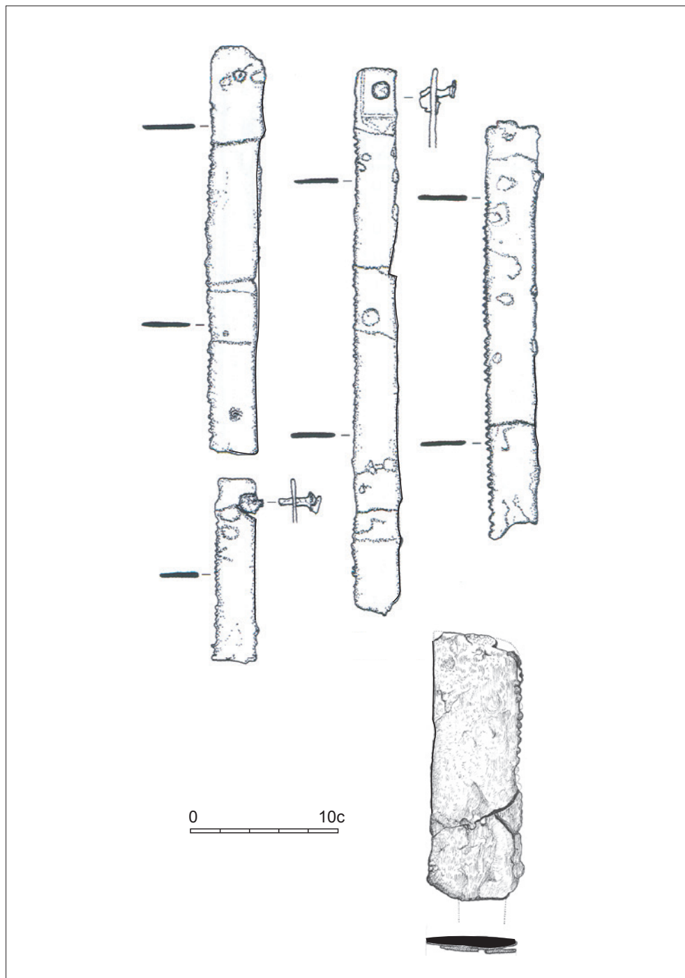
176. Conjunt de serres de Mas Castellar (Pontós), datat cap al 190 aC.
