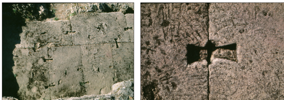
58. Panisars, trofeu de Pompeu. Els grans carreus del mur perimetral s'unien amb grapes de fusta en forma de cua d'oreneta per assegurar-ne l'estabilitat. Amb el pas del temps van desaparèixer.
