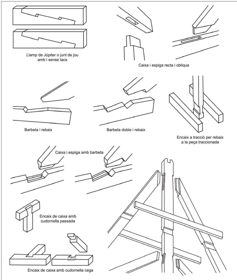
178. Principals tipus d'encaixos i unions en fusta utilitzats en els sistemes tradicionals de construcció d'estructures amb aquest material.
