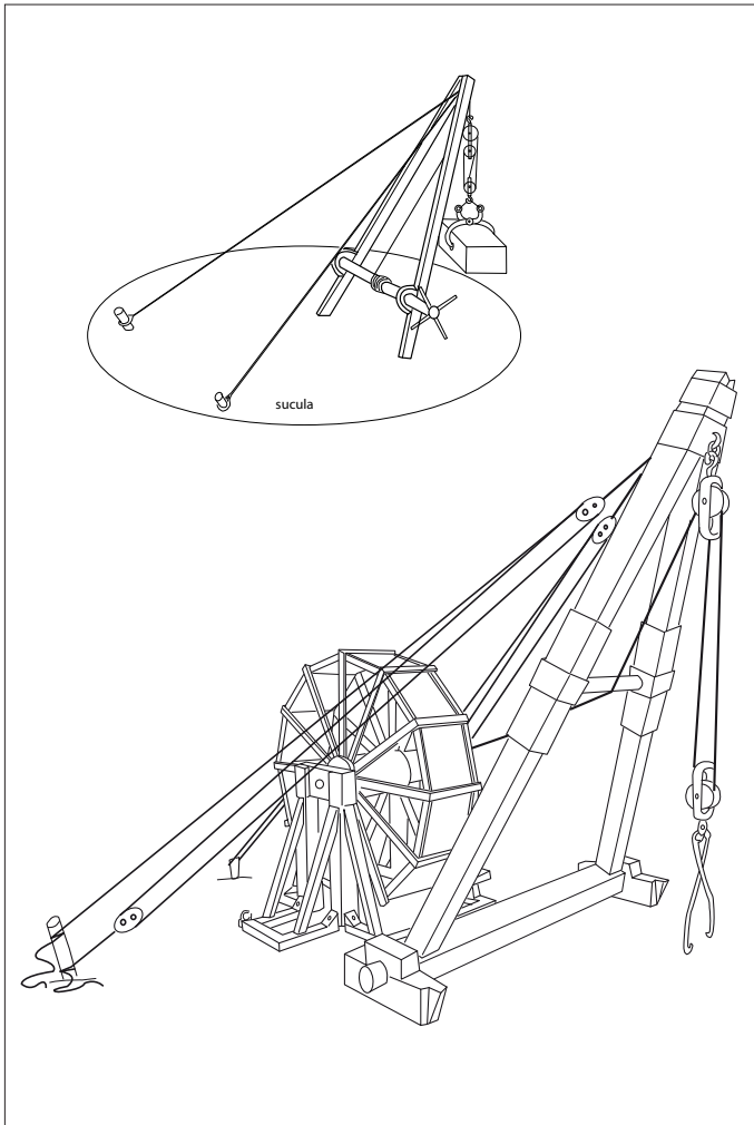
53. L'ús de grues degué ser usual, com bé ens explica Vitruvi, en el transport i a l'hora d'edificar.
