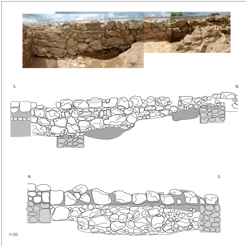
81. Mas Gusó. Composició. Mur de pedra seca lligada amb fang.
