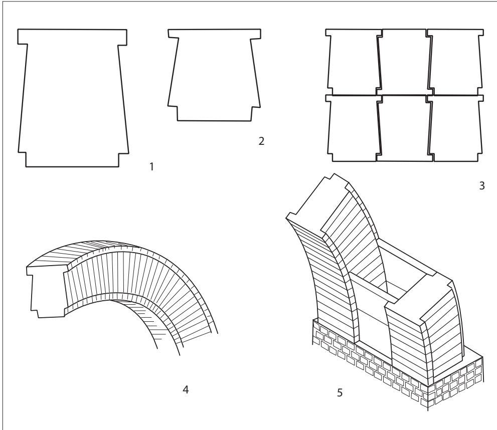
35. Exemple de la fabricació i ús d'un tipus concret de rajol utilitzat per obrar les concamerationes (espais compartimentats dels murs de les sales calentes d'un balneum per on circulava l'aire calent).
