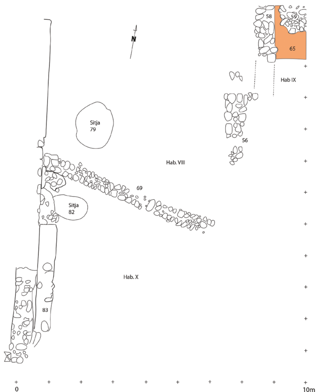
Figura 28. La Quintana. Planta del sector A, amb les «suposades habitacions» HVIII, HIX i HX (1983).
