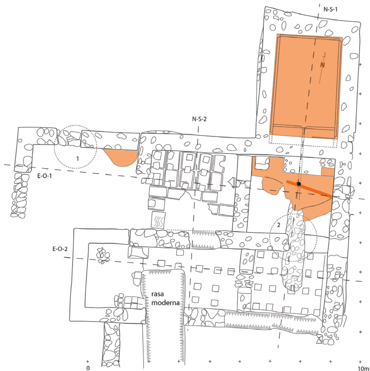
Figura 11. La Quintana. Planta general balneum . S'assenyalen els espais amb sòls d' opus signinum i la presència de dues sitges baix-republicanes preexistents.
