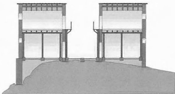
Fig 50. Edifici I. Secció transversal (nord-sud) (fase II).
