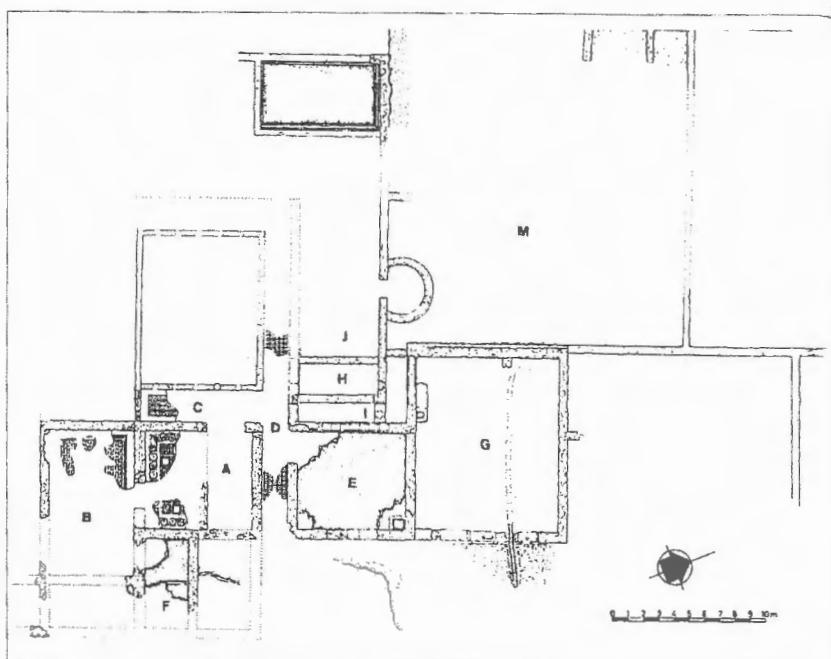
Fig 106. Vil·la del Pla de l'Horta (Sarrià de Ter). Planta general.
