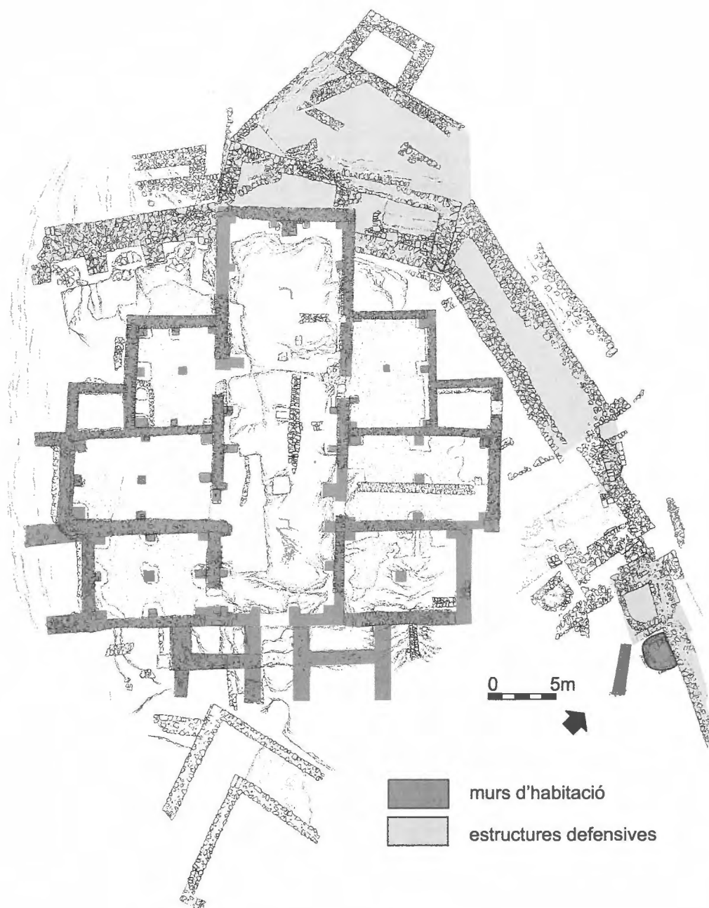
Fig 49. Fase II. Planta general.
