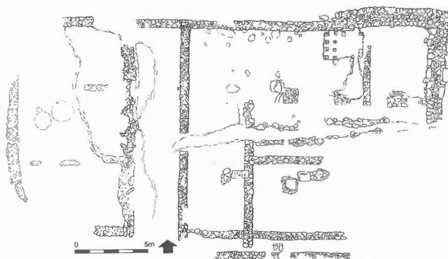
Fig 125. La mansio de Summum Pyrenaeum . Planta.
