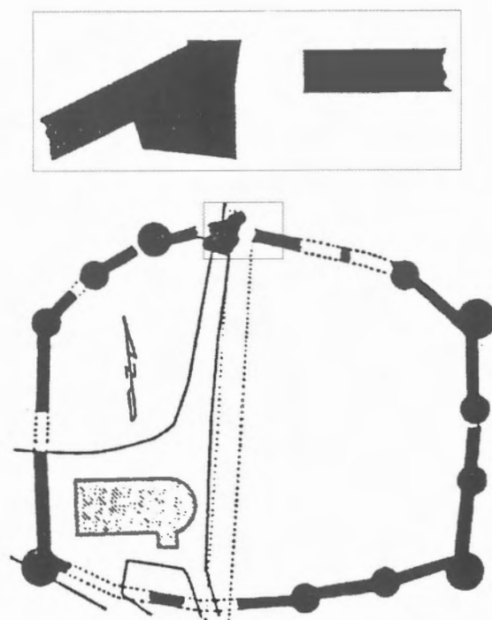
Fig 15. Planta de les defenses baiximperials de Neumagen i detall de la porta (segons Lander, 1984).
