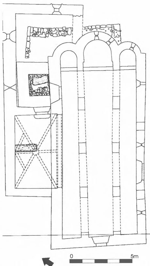
Fig 56. Edifici IV dins de les estructures de l'esglesiola actual.
