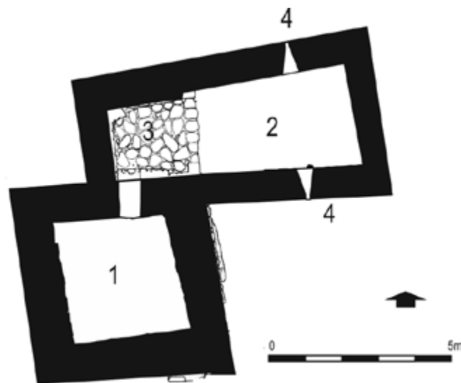
Figura 31. Planta baixa de la torre i el reducte del mas Llorens. 1) Torre, 2) reducte, 3) paviment de lloses i 4) espitlleres.
