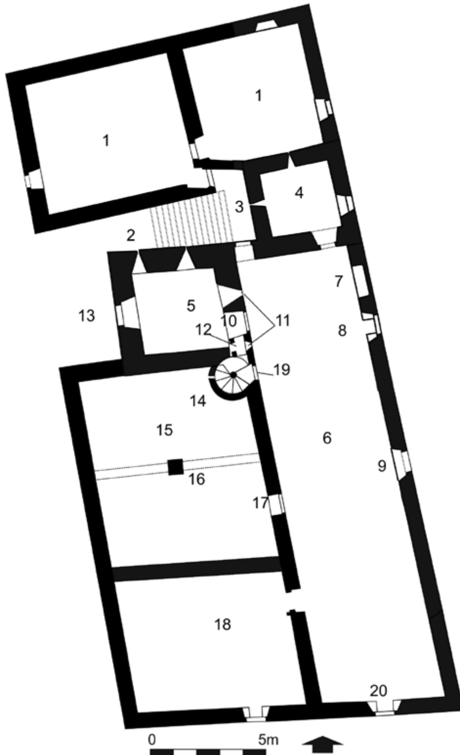
Figura 29. Planta primera restituïda de la part coneguda del mas Llorens al segle XVI: 1) àmbit nord; avui només se'n conserven les façanes, 2) escala principal, 3) replà, 4) tram superior de l'antic reducte, 5) torre, 6) sala, 7) tinell, 8 i 9) finestres d'arc conopial, 10) porta que comunica la sala amb la torre, 11) troneres dobles, 12) defensa de l'espitllera doble sud, 13) antiga porta de la torre, 14) escala de cargol en forma de torrella, 15) pati, 16) pilar de pedra de dues plantes, 17) porta de permòdols, 18) estança sud occidental, 19) porta d'accés a l'escala de cargol des de la sala cambra sud i 20) finestra de la cambra sud.
