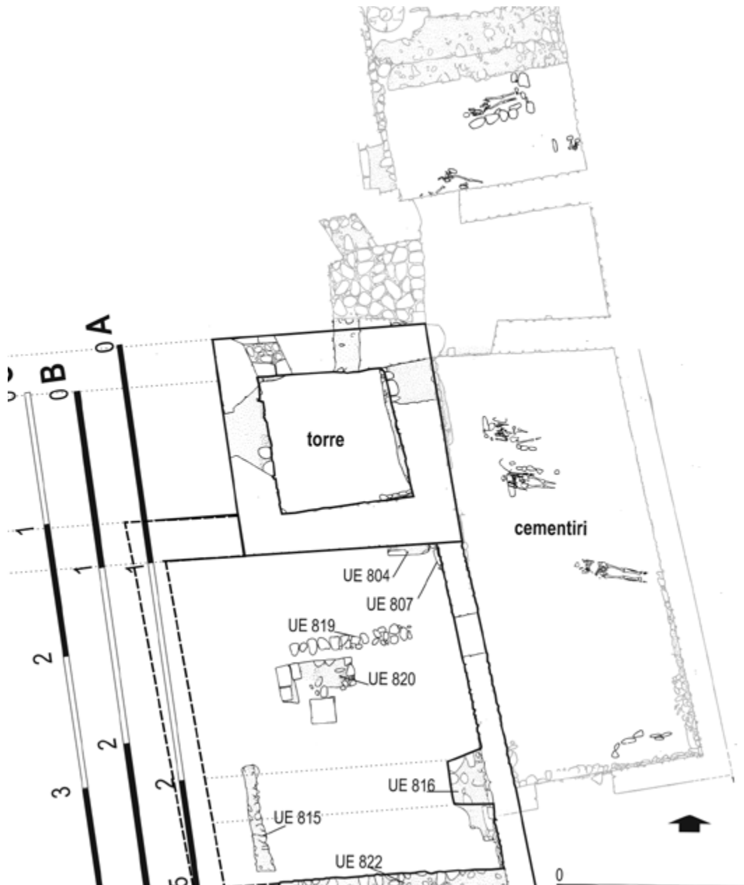
Figura 13. Planta dels elements i estructures relacionades amb la casa forta medieval del mas Llorens. S'endevina la disposició i la implantació dels àmbits a partir d'una modulació predeterminada. Les tres escales gràfiques situades a l'esquerra permeten argumentar-ne algunes a partir de mesures derivades de la planta de la torre : A) la unitat de mesura correspon a la longitud de la façana, B) la unitat comprèn la llum interior més el gruix d'un mur de façana i C) la unitat correspon a la llargada de l'espai interior.
