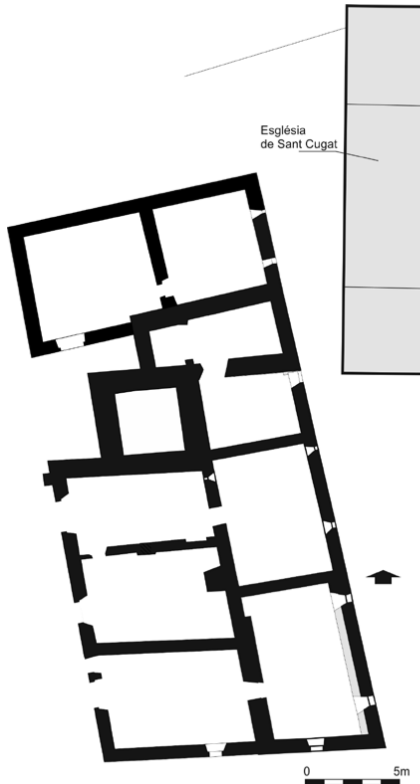
Figura 79. Plànol de la planta baixa del mas Llorens al segle XVII.
