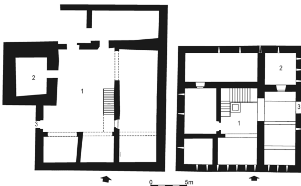
Figura 18. Plantes de cases fortes; a l'esquerra, el mas Sitjar i a la dreta, la torre Ferrana de Montfullà. Les proporcions i distribucions són similars i defineixen un recinte quadrat amb un pati central (núm. 1) on hi trobem la cisterna i l'escala d'accés a la planta noble, presidida per la sala. La torre (núm. 2) domina la façana principal i se situa a prop de la porta d'entrada al recinte (núm. 3).
