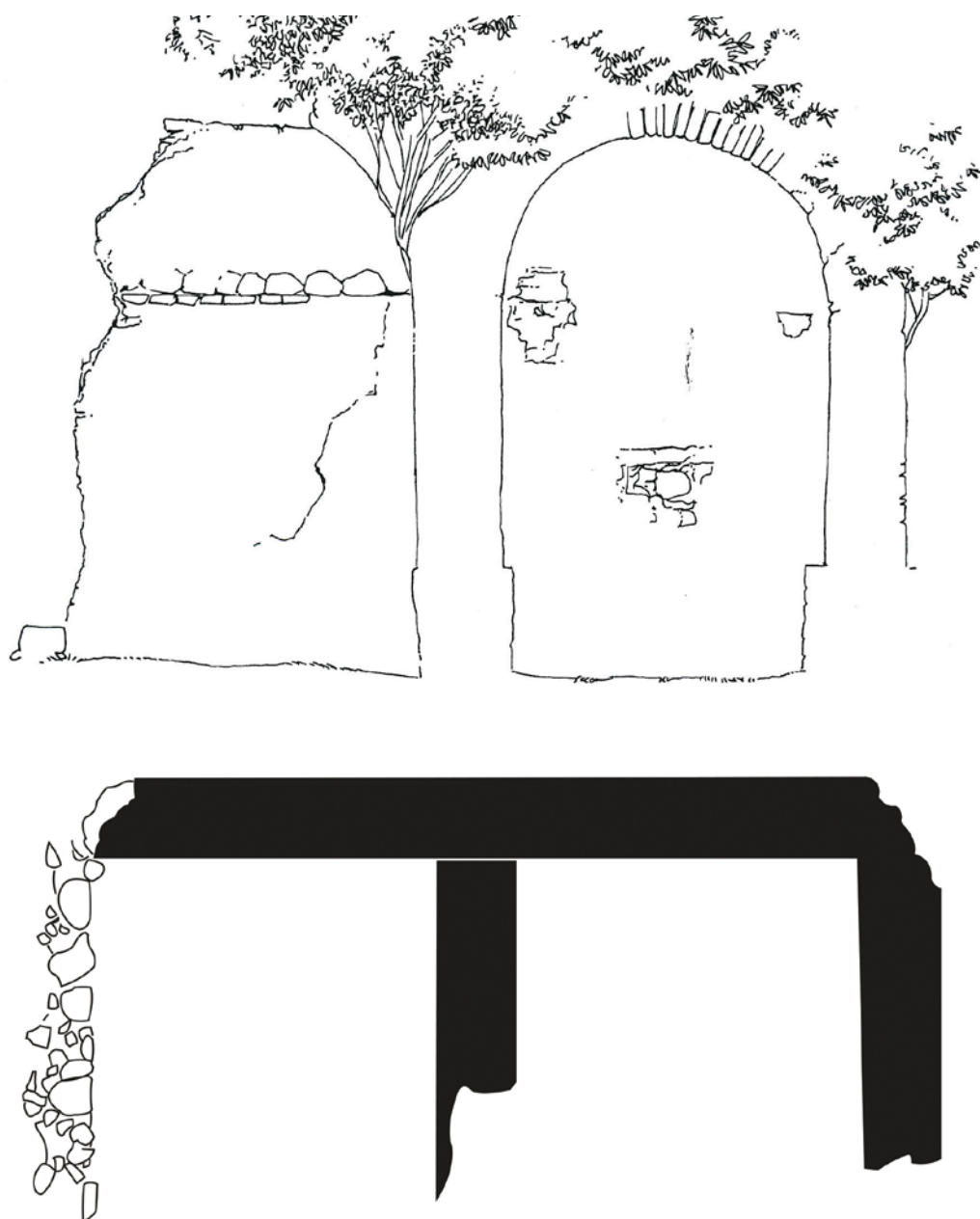
Figura 3. Cavorca II (o can Cavorca). Planta i alçat interior.
