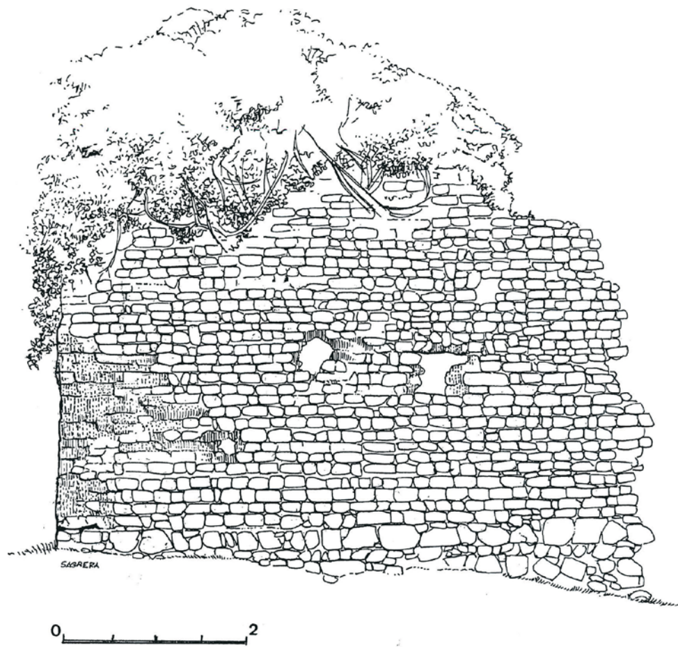
Figura 4. Cavorca II (o can Cavorca). Alçat exterior del mur occidental.
