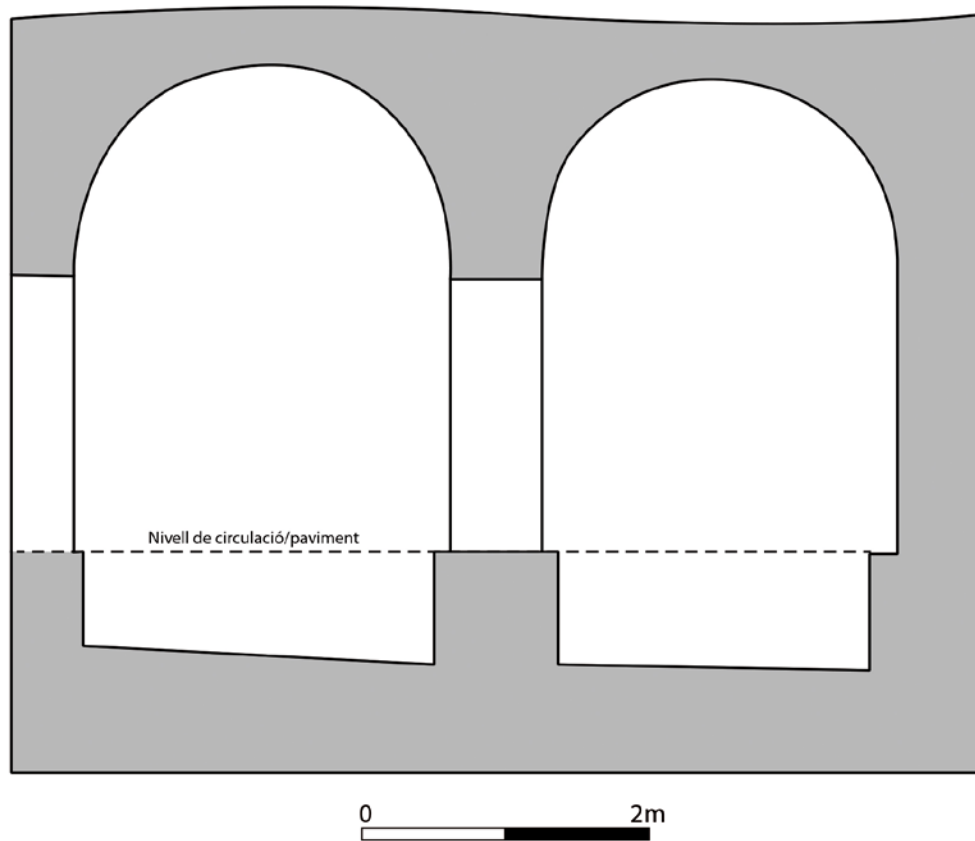
Figura 9. Cavorca II (o can Cavorca). Secció longitudinal amb la restitució del sòl interior de l'edifici.
