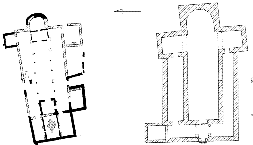
fig. 27.- A dalt, planta del temple del Tolmo de Minateda (Hellín, Albacete) i a baix, del de Recópolis (Zorita de los Canes, Guadalajara).
