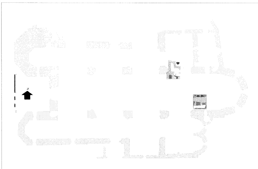
fig. 9.- Sant Feliu de Girona. Planta actual del temple amb la situació dels sondeigs realitzats l'any 2010.
