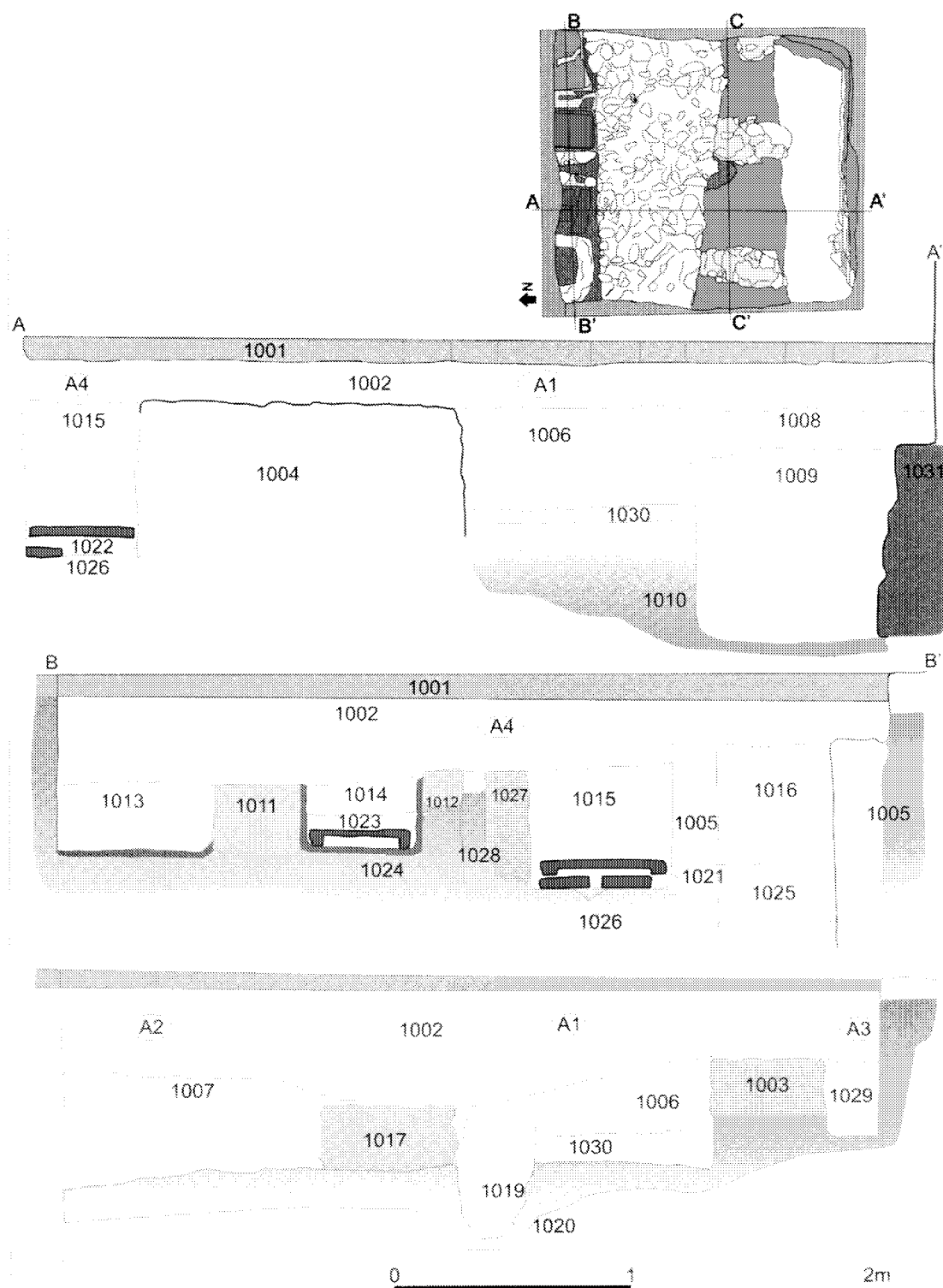
fig. 11.- Sant Feliu de Girona. Sondage 1. Seccions.
