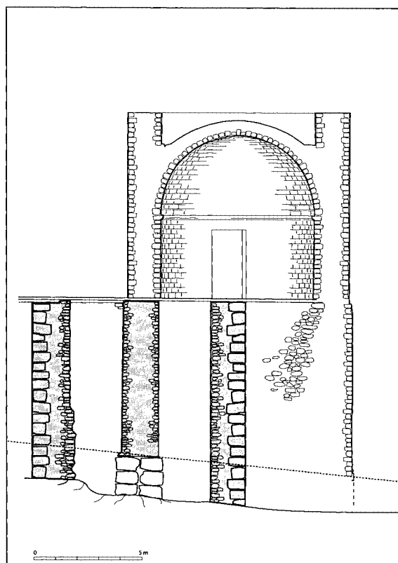
Figura 4. Secció del sector de ponent de Sobreportes amb indicació de les torres bessones tetràriques, la muralla i la torre cilíndrica baixmedieval
