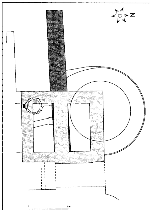
Figura 3. Planta del sector occidental de Sobreportes, amb indicació de les torres romanes bessones i la muralla
