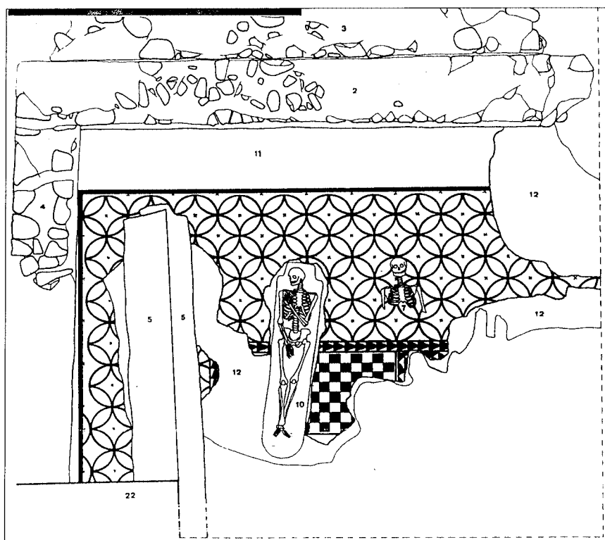
FIGURA 4 B. Sant Pere de Montfullà. Plantes finals. Excavació 1987 (segons Nieto, Puig i Merino, 1989).
