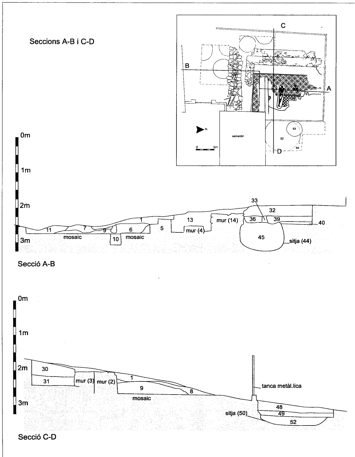
FIGURA 66. Excavació de 2002. Seccions generals.
