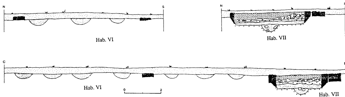
Fig. 6- Seccions nord-sud i oest-est de la nau de dolia (Hab. VI) que conté en el seu angle sud-est el dipòsit revestit d' opus signinum (Hab. VII).
