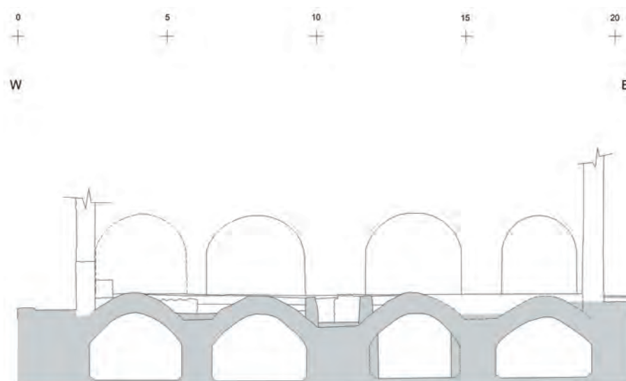
Figura 15. Cubelles. Secció de les cisternes bastides el c. 200 dC, amb indicació dels arcs del c. 360.
