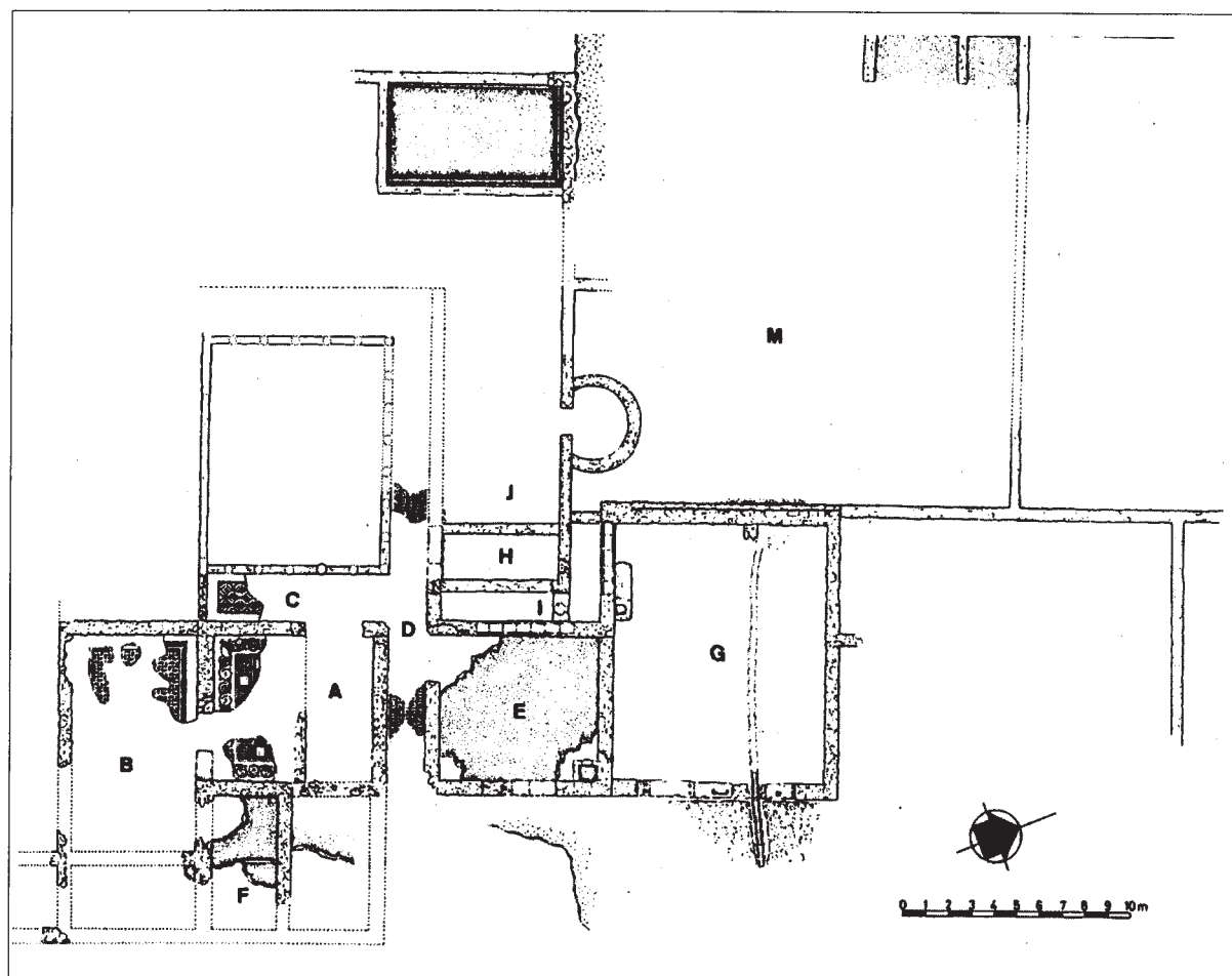
Figura 5. Detall de la pars urbana de la vil·la del Pla de l'Horta en època severiana.
