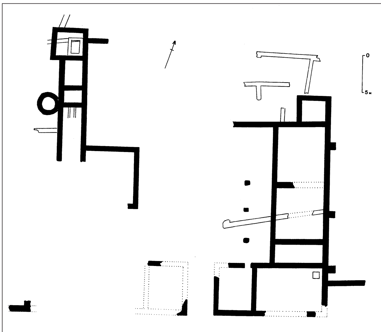
Figura 4. Planta de la darrera fase constructiva de la vil·la de Mas Gusó
