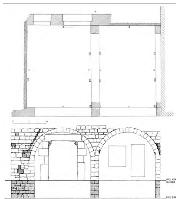
Figura 2. Planta i un dels alçats elaborats el 1987.
