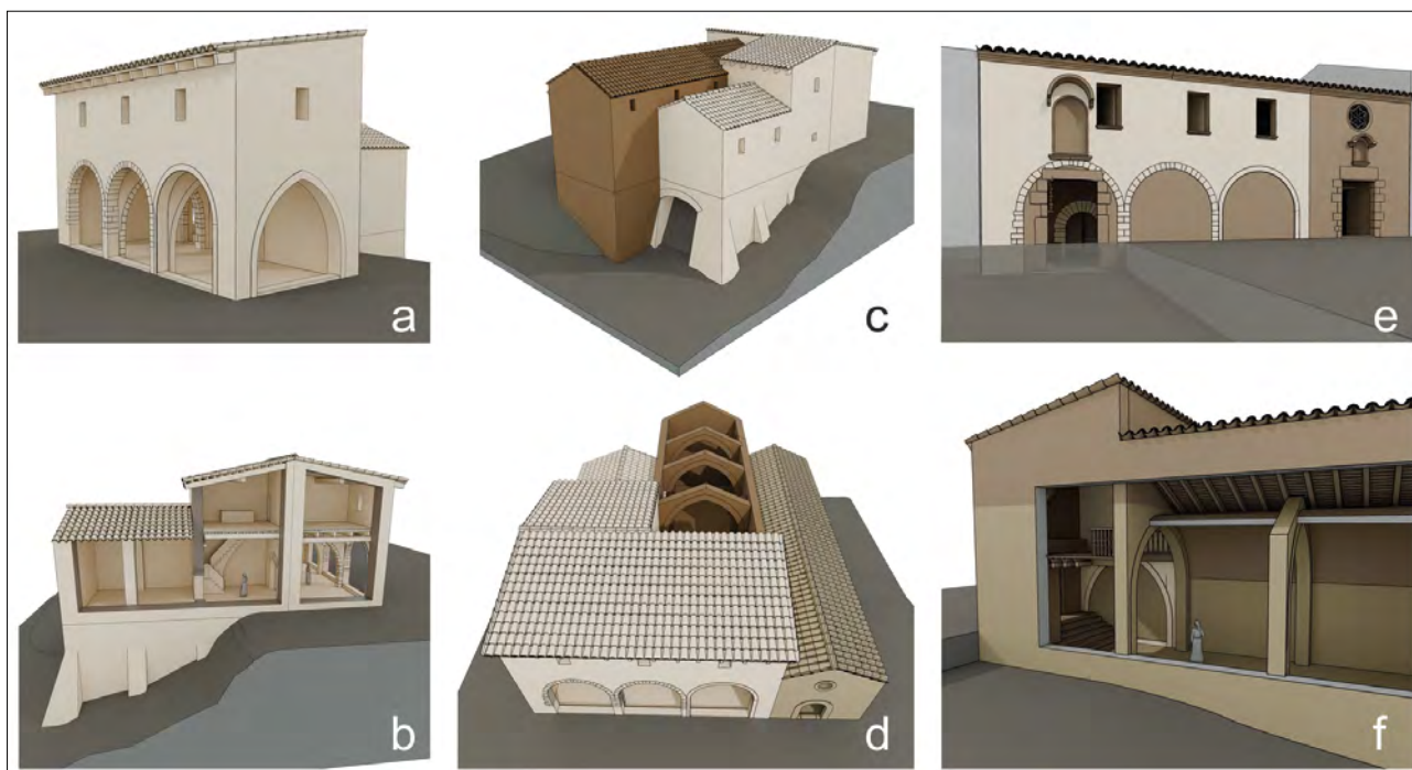
Figura 6. Vistes del model tridimensional de l'hospital i la capella de Sant Joan: Imatge de la façana, amb el porxo i la segona planta (a) i tall lateral que ens mostra l'interior de la crugia esquerra i la planta superior sobre el porxo, amb l'escala d'accés (b). En color marró fosc, volum exterior (c) i disposició dels arcs de diafragma de la crugia dreta amb la capella de Sant Joan, adossada el 1310 (d). Façana del conjunt de l'hospital i la capella, amb les modificacions del segle XVIII un cop elevada la rasant del carrer (e) i vista de l'interior de la capella, amb la incorporació del cor i la falsa volta entre els arcs de diafragma (f).
