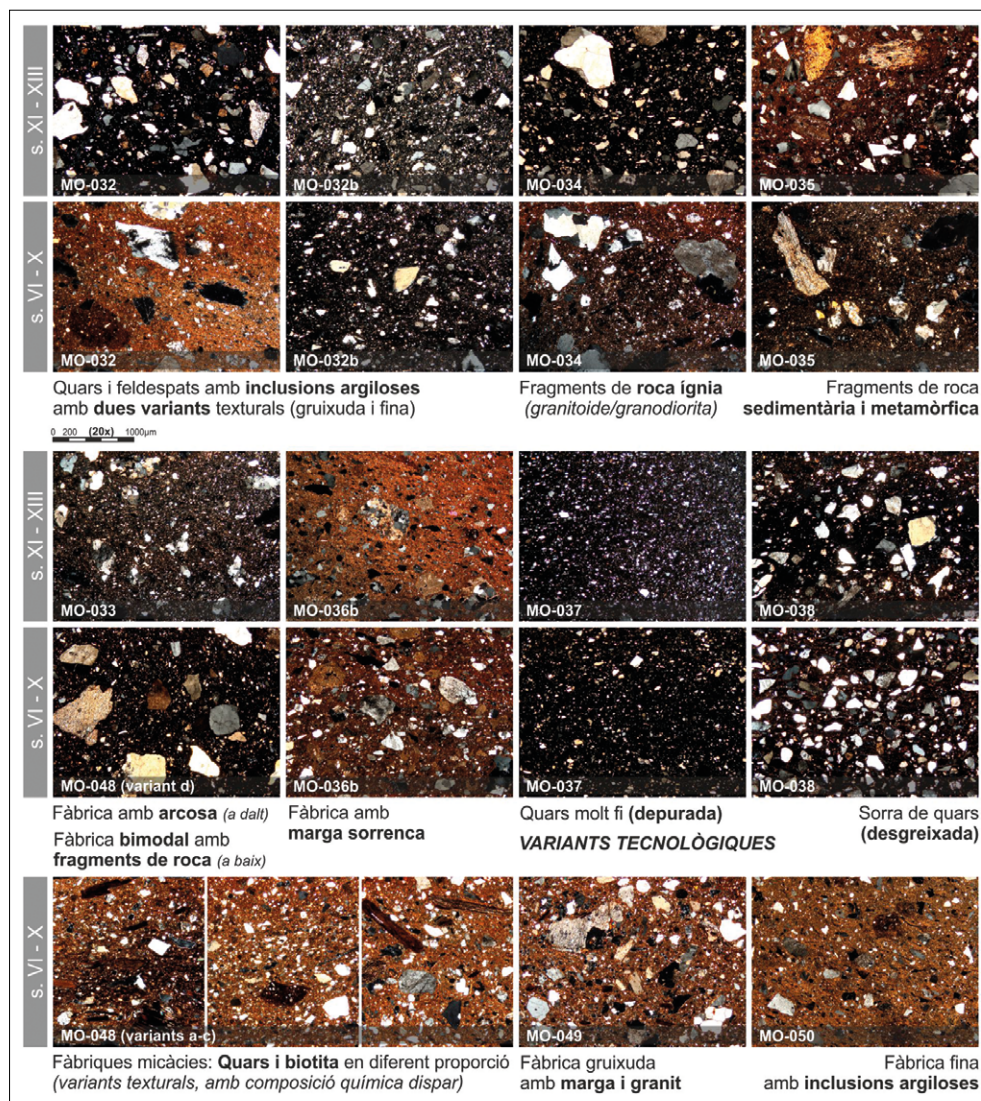
Figura 5. Quadre-resum gràfic de les principals fàbriques identificades, en relació amb les diferents fases estudiades. Totes les micrografies han estat preses amb nicols creuats i representen un camp de visió de 6 mm.
