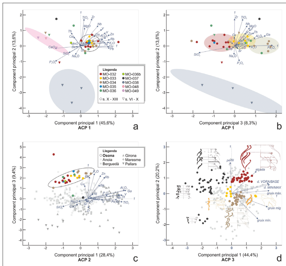
Figura 6. Gràfiques de doble entrada resultants de les anàlisis de components principals (ACP) practicades en funció de les dades químiques del material estudiat (a i b), dels materials de l'Esquerda comparats amb altres produccions catalanes (c) i de les dades morfomètriques del conjunt de ceràmica grisa de l'Esquerda (d), sempre interpretades en funció de les fàbriques identificades.
