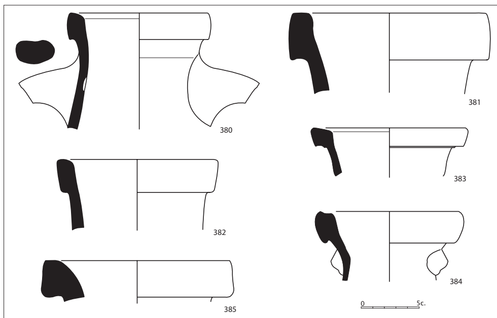
Figura 2.89. Àmfores Keay 59.
