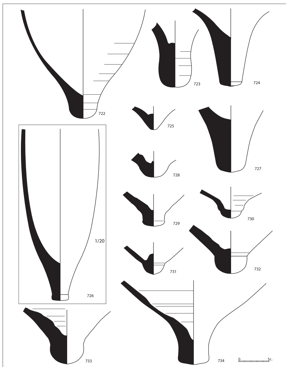
Figura 2.142. Pivots d'àmfores de formes indeterminades.
