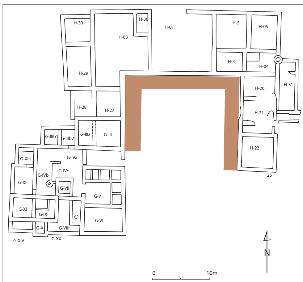
Figura 2.152. Ciutadella de Roses. Planta general de l'«Edifici A» on restituïm el porticat que envoltava i definia el pati G-II.
