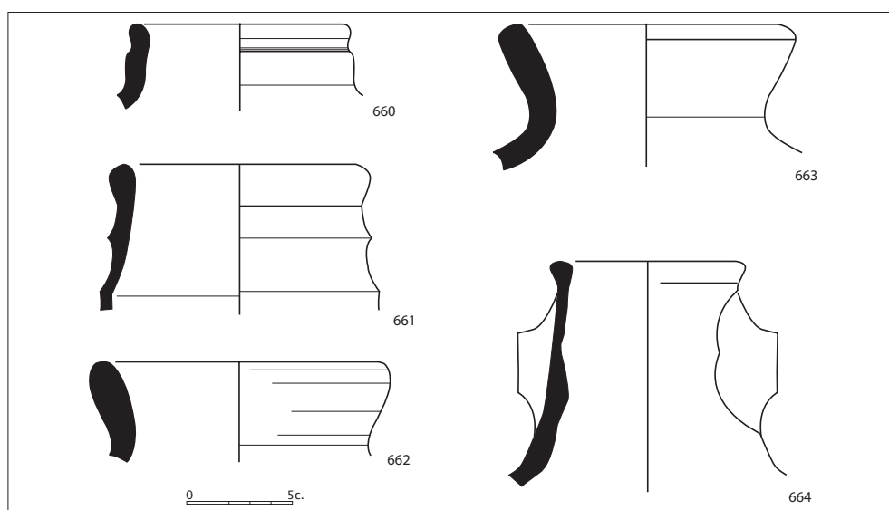
Figura 2.135. Àmfores LRA 5-6; àmfora LRA 15.
