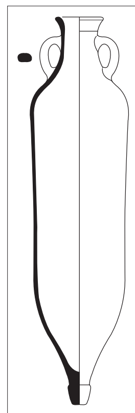
Figura 2.42. Forma tipus. Àmfora tipus Africana III A.
