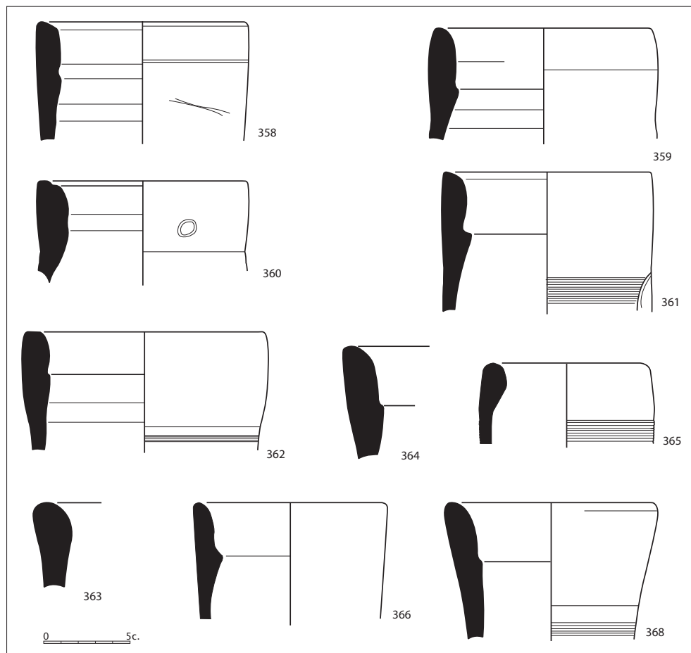
Figura 2.83. Àmfores Keay 55.
