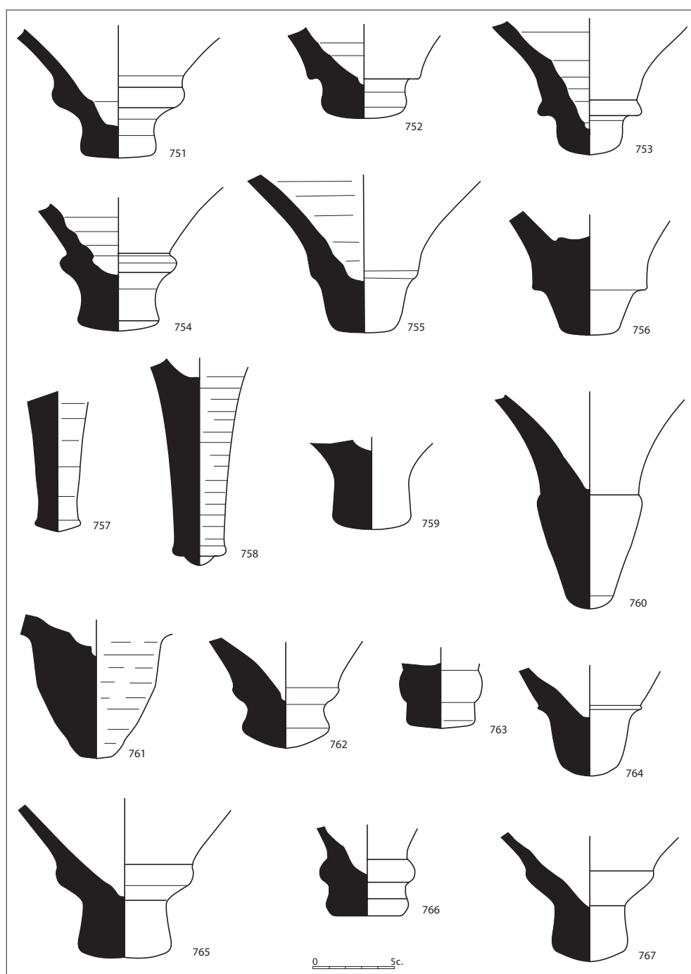
Figura 2.144. Pivots d'àmfores de formes indeterminades.
