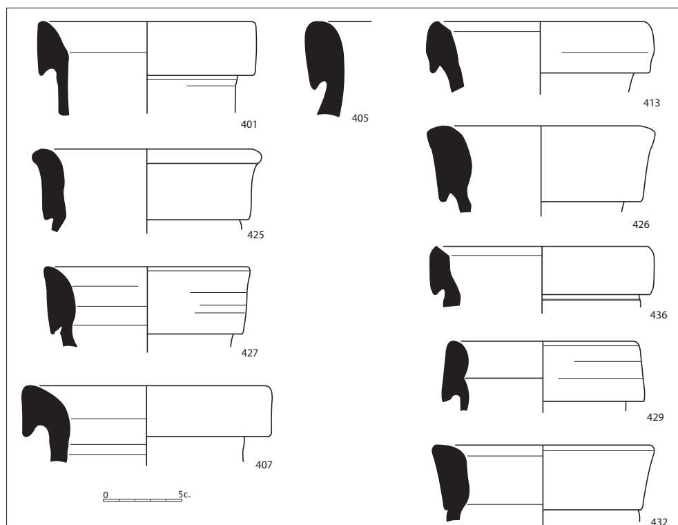
Figura 2.96. Àmfores Keay 61.
