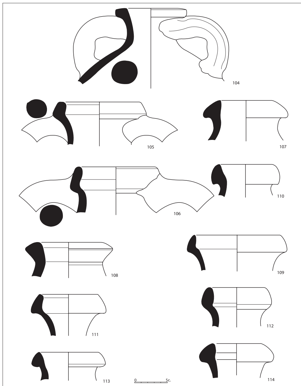
Figura 2.31. Àmfores Keay 13 A.
