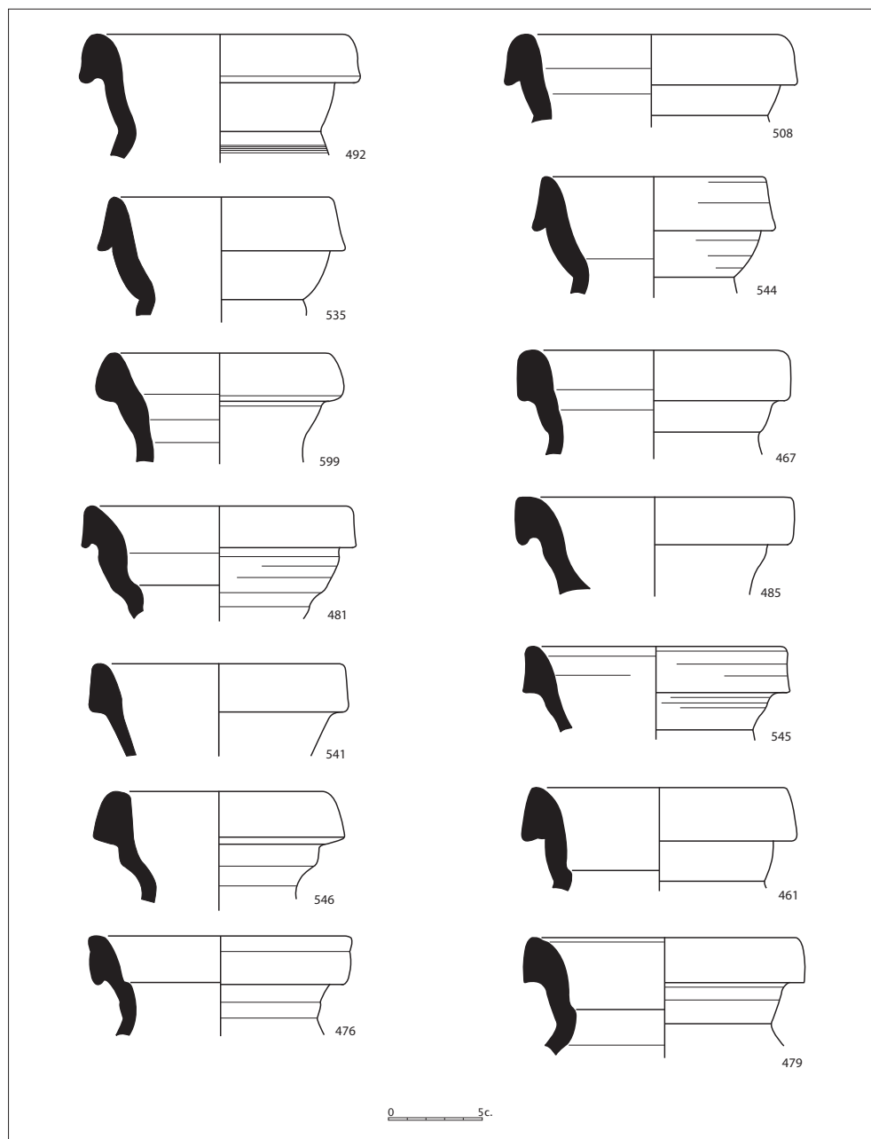
Figura 2.103. Àmfores Keay 62, formes varies (veure catàleg).
