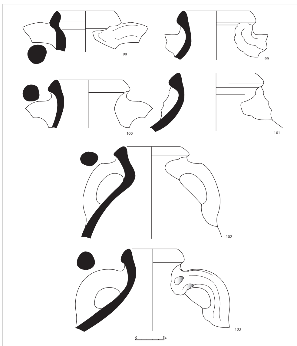
Figura 2.30. Àmfores Keay 13 A.
