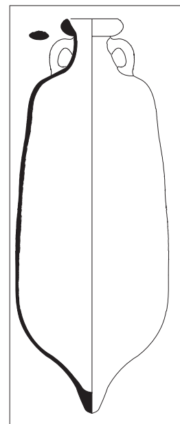
Figura 2.13. Forma tipus. Àmfora Pupput T700.
