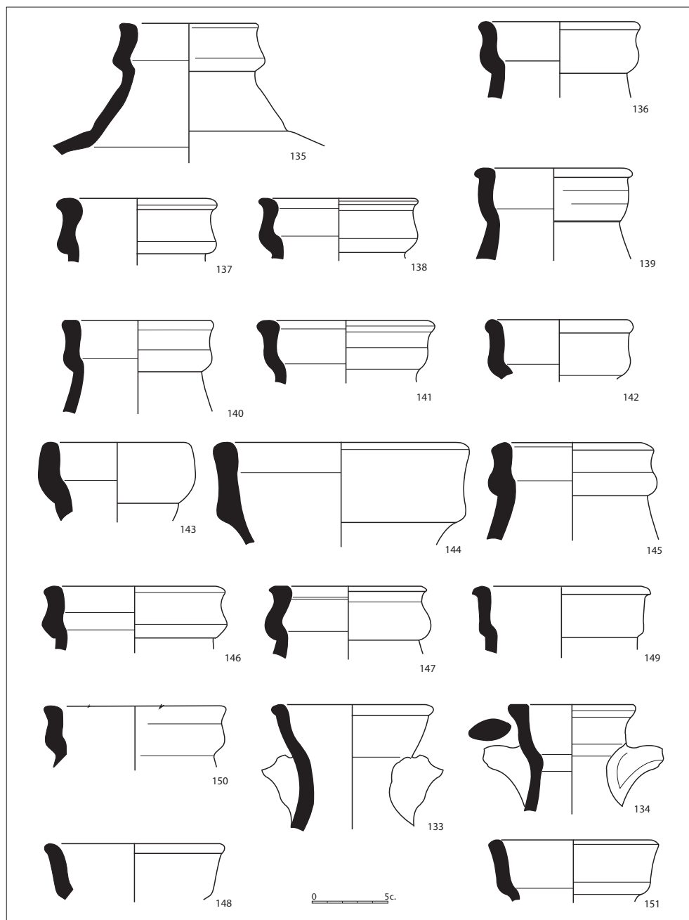
Figura 2.37. Àmfores Keay 19 A-B I Keay 68/91 o Algarve 1.
