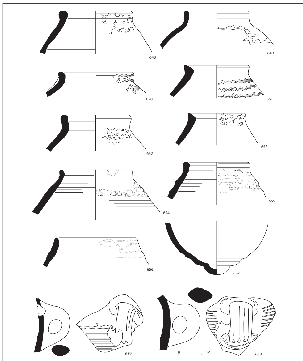
Figura 2.133. Àmfores LRA 4.
