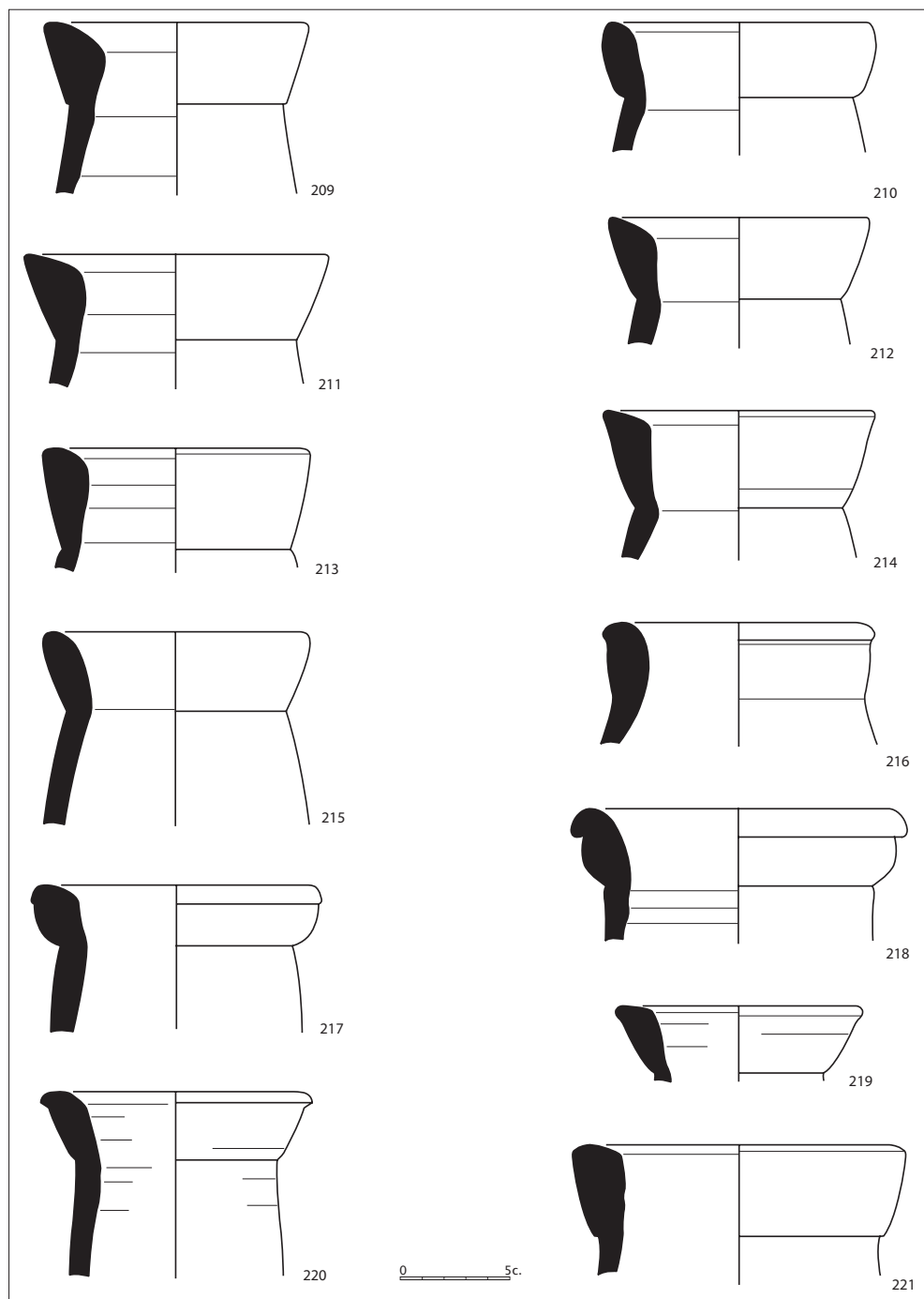
Figura 2.53. Àmfores Keay 25 B.
