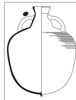
Figura 2.128. Forma tipus. Model genèric de l'àmfora LRA 2.
