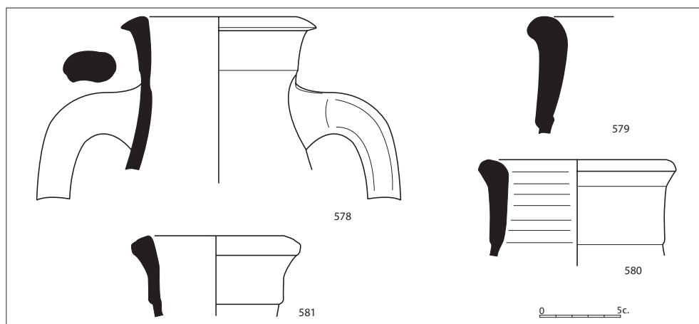
Figura 2.112. Àmfores Keay 8 A i 8 B.
