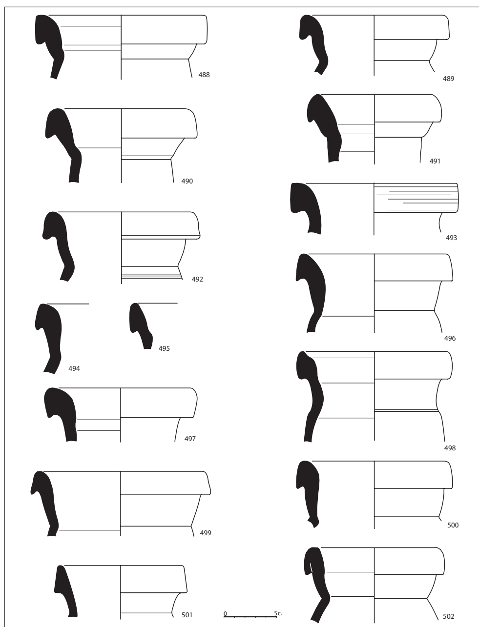
Figura 2.102. Àmfores Keay 62.
