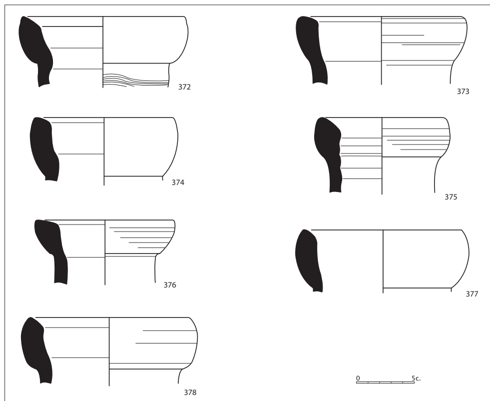
Figura 2.87. Àmfores Keay 57.
