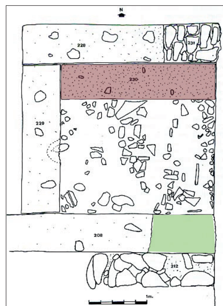
Figura 2.166. Ciutadella de Roses. «Edifici A», planta de detall de l'habitació G-XIII, el vestidor del balneum alt-imperial, amb la porta al costat meridional i un banc corregut d'obra, al fons (nord), remarcats amb colors diferenciats.
