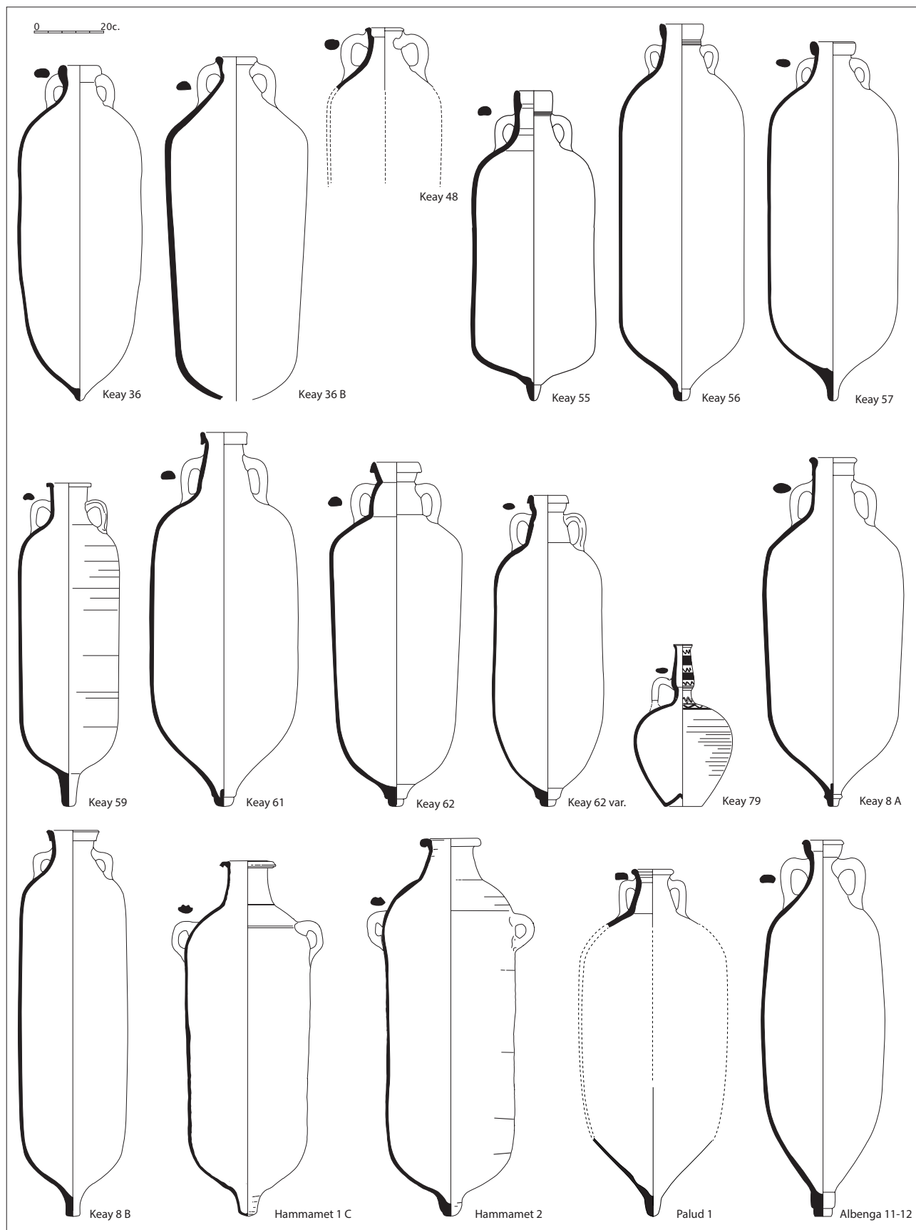
Figura 3.3 . Tipologia general de les àmfores descrites en aquest treball (Keay 36 a Albenga 11-12).
