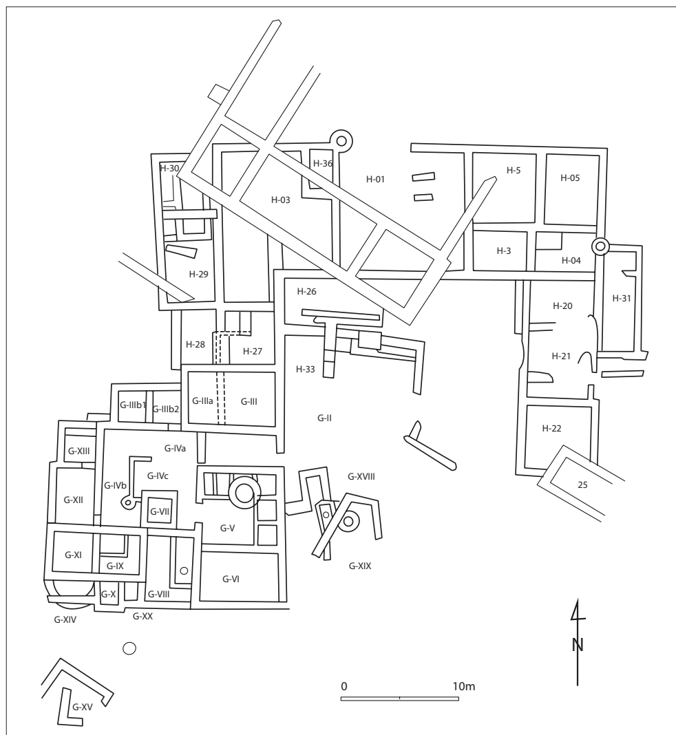
Figura 2.149. Ciutadella de Roses. Planta de l'«Edifici A», tot remarcant els sectors H i G, indicant el nom atorgat a cada una de les estances.
