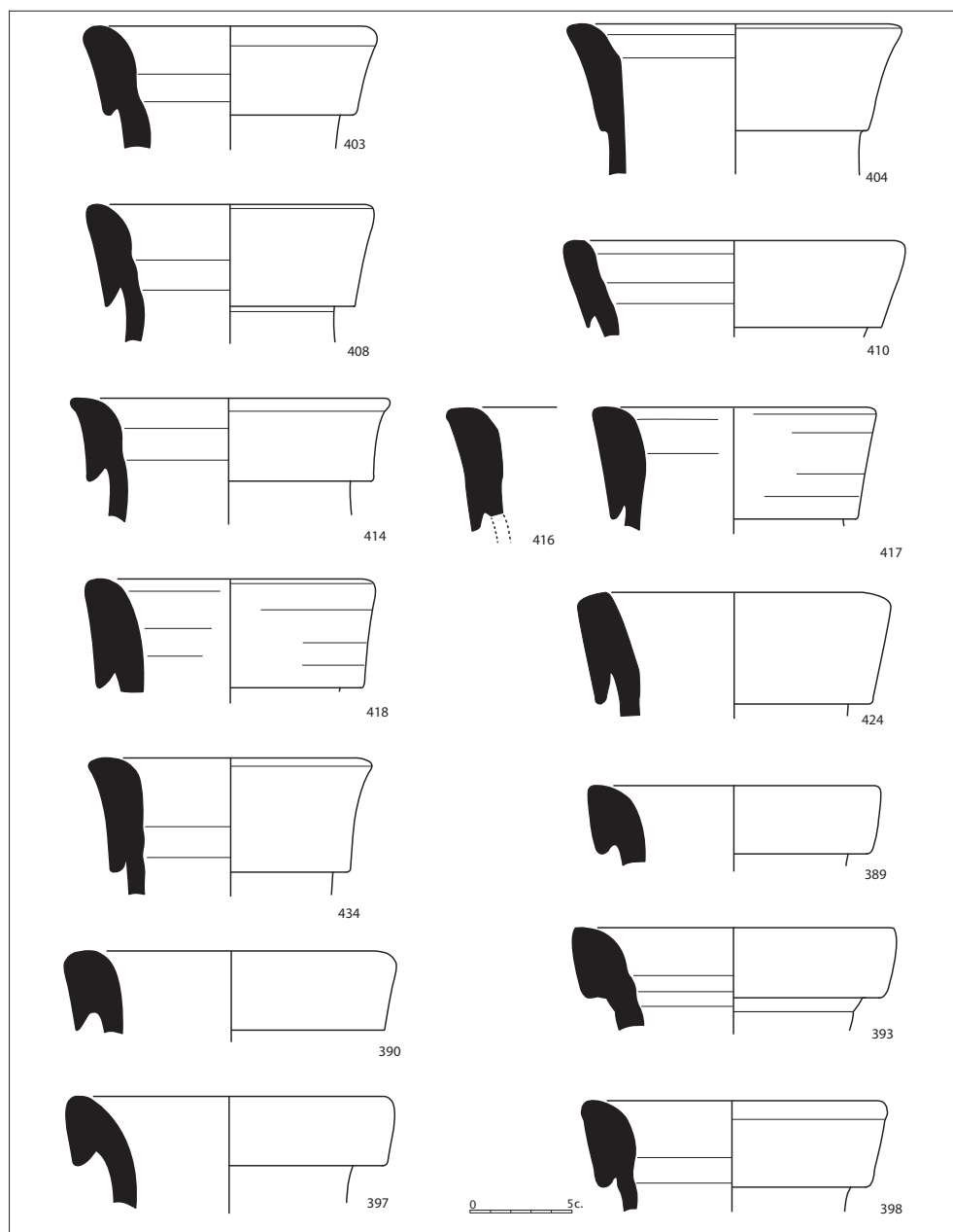
Figura 2.92. Forma tipus. Àmfora tipus Keay 61.
