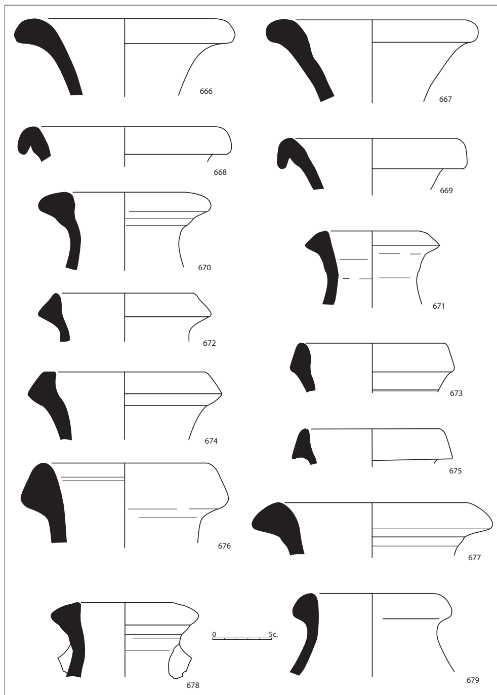
Figura 2.138. Àmfores de tipologia indeterminada.
