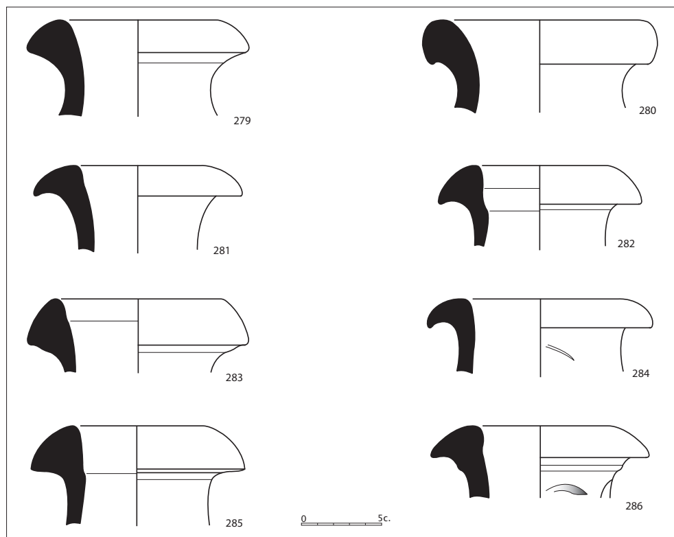
Figura 2.69. Àmfores Keay 35 B.
