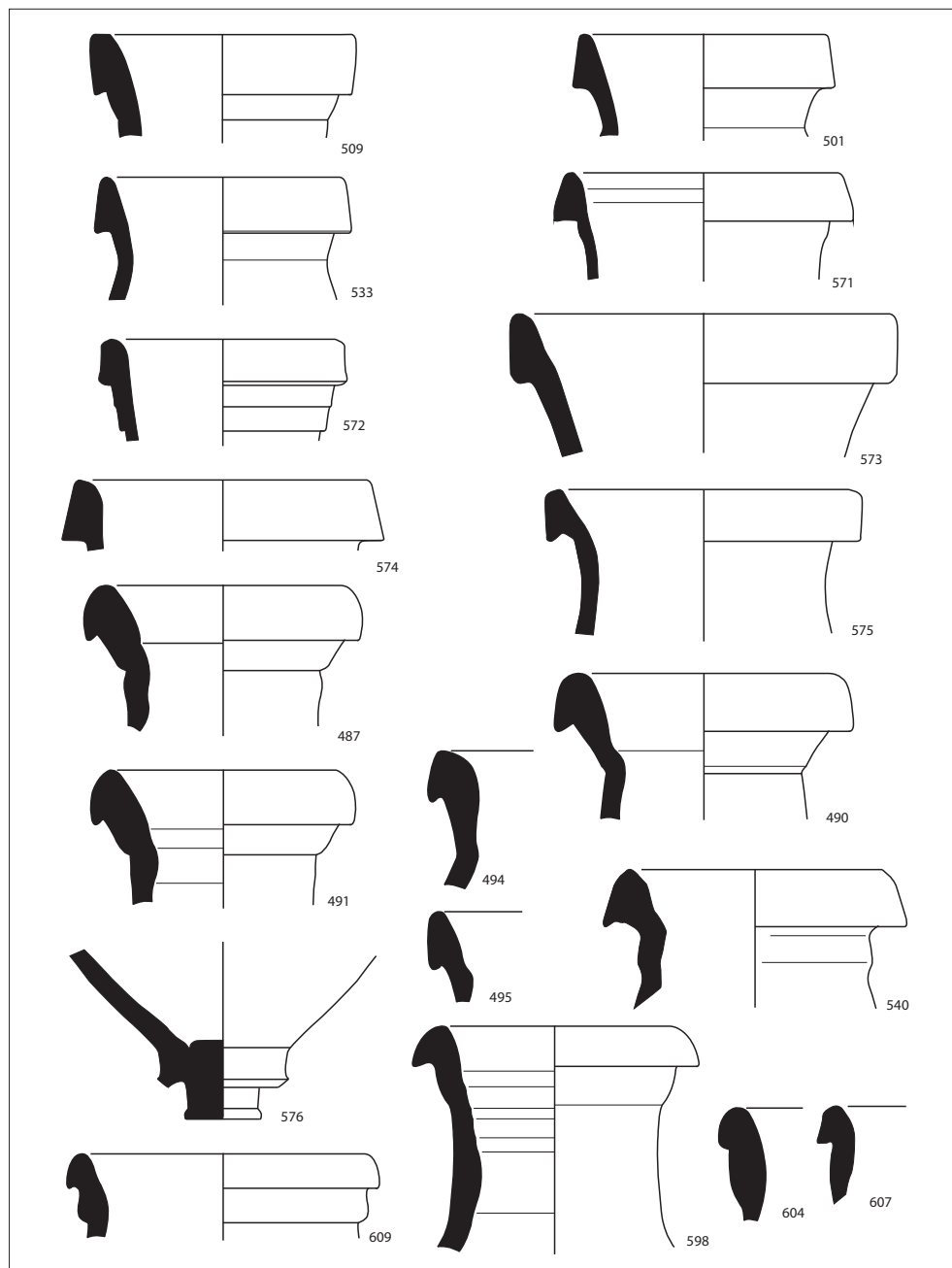
Figura 2.108. Altres variants de l'àmfora Keay 62.
