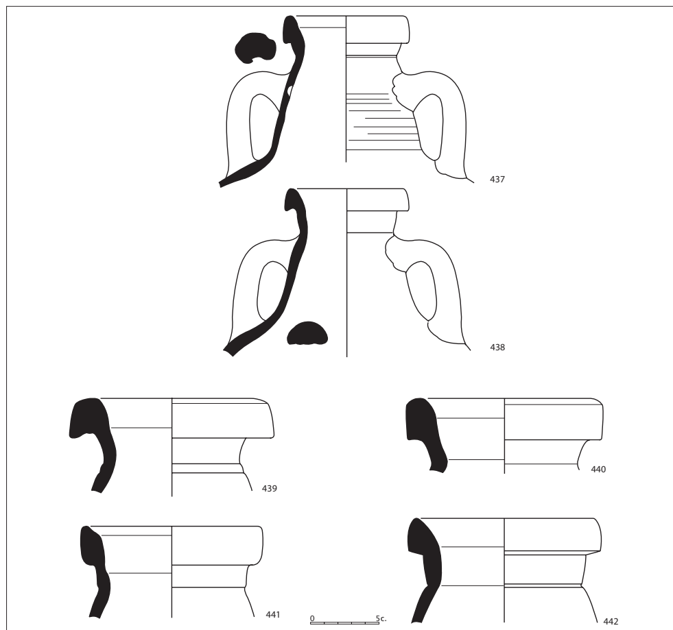
Figura 2.98. Àmfores Keay 62 A.
