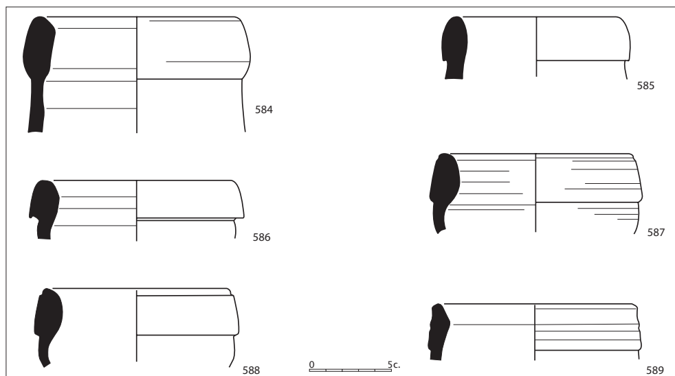
Figura 2.115. Àmfores Keay 92.
