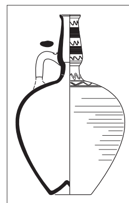
Figura 2.109. Forma tipus. Àmfora tipus Keay 79.
