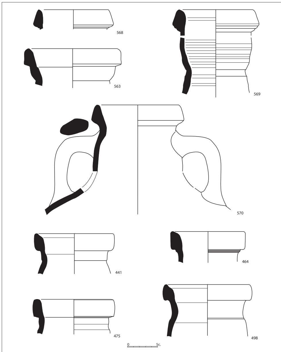
Figura 2.107. Àmfores Keay 62, formes variades (veure catàleg).
