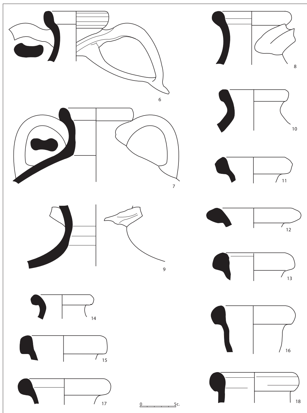
Figura 2.5. Àmfores G-4.
