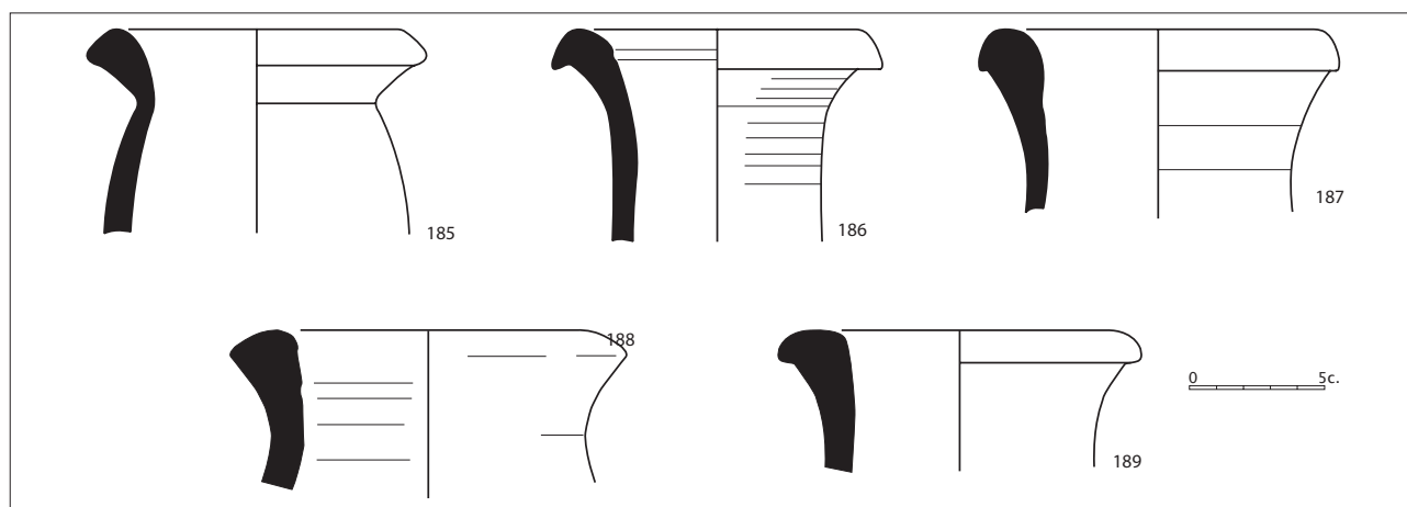
Figura 2.49. Àmfores Keay 25.
