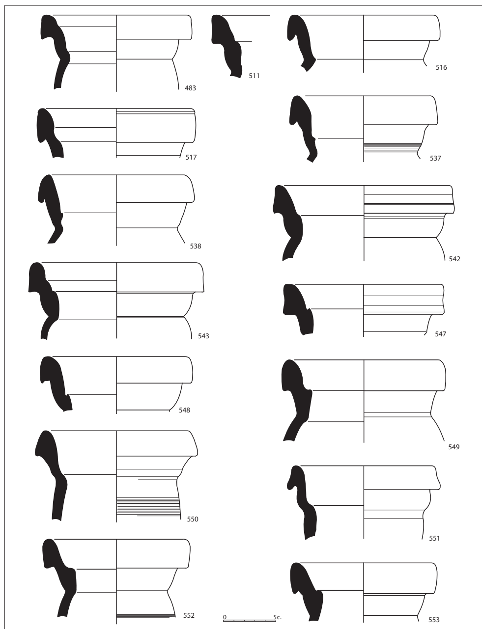
Figura 2.104. Àmfores Keay 62 D.
