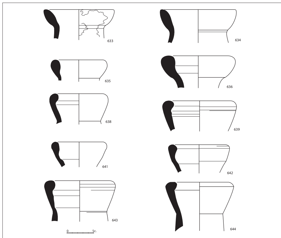
Figura 2.129. Àmfores LRA 2A.
