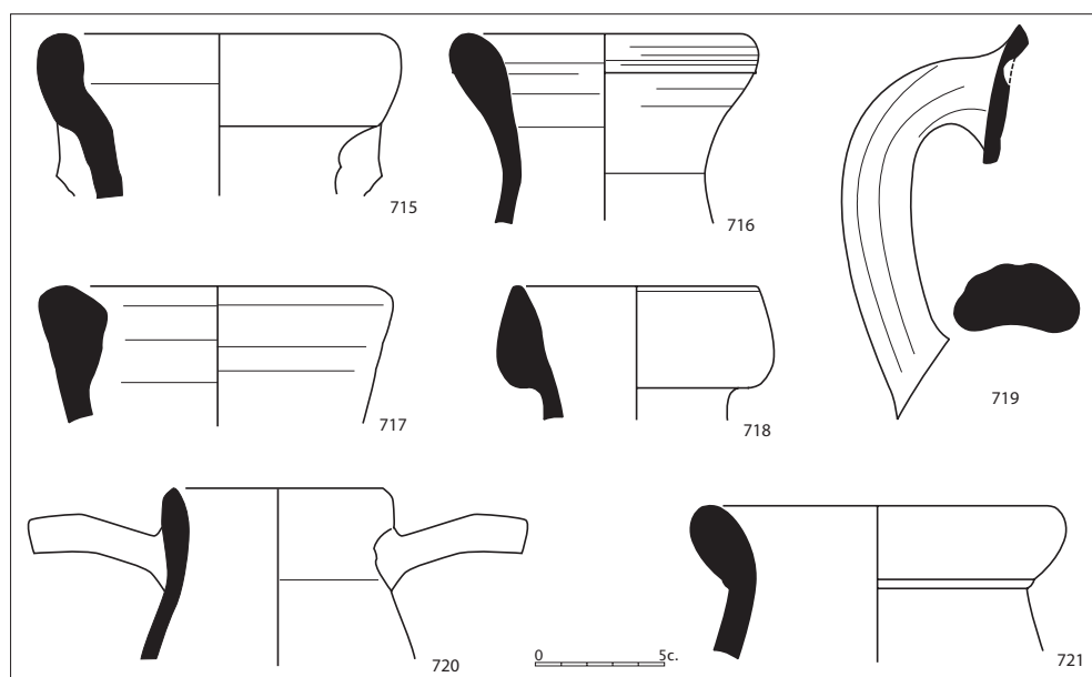
Figura 2.141. Àmfores de formes indeterminades.
