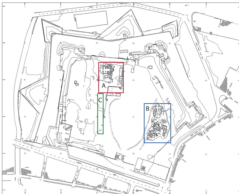
Figura 1.4. Planta general de la ciutadella de Roses on s'assenyalen els llocs d'excavació i treball entre 1945 i 1985. A) sector de Santa Maria, B) «Barri hel·lenístic» i «Edifici A», C) Situació generals d'uns sondejós i rases efectuats el 1961 i 1963.
