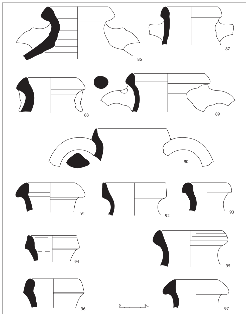
Figura 2.29. Àmfores Keay 13 A.
