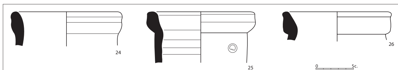
Figura 2.8. Àmfores Tripolitana II.
