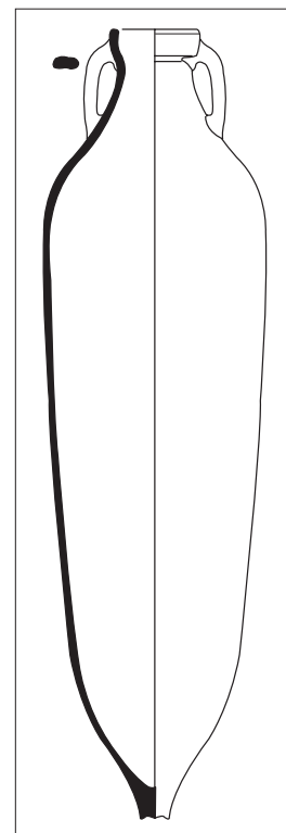
Figura 2.61. Forma tipus. Àmfora tipus Keay 28.
