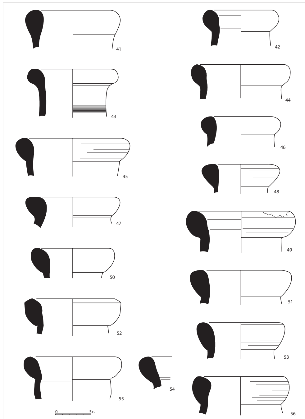
Figura 2.18. Àmfores Africana II A.
