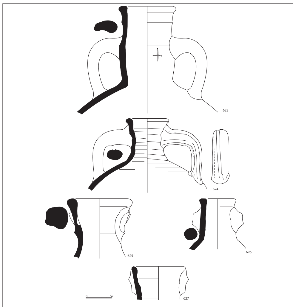
Figura 2.126. Àmfores LRA 1.
