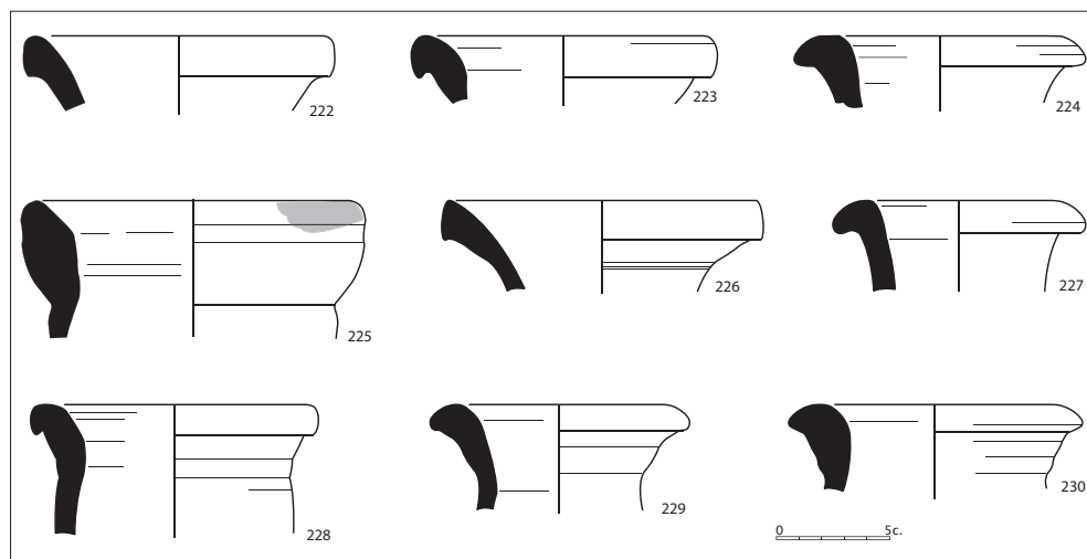
Figura 2.55. Àmfores Keay 25 C; àmfora Keay 25 D; àmfores Keay 25 E; àmfora Keay 25 F; àmfores Keay 25 L.
