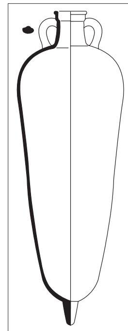
Figura 2.36. Forma tipus. Tipus genèric de l'àmfora Keay 19 A-B.
