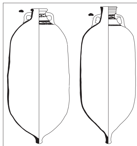
Figura 2.120. Forma tipus. Àmfora tipus Sidi Jdidi 1 i 2.
