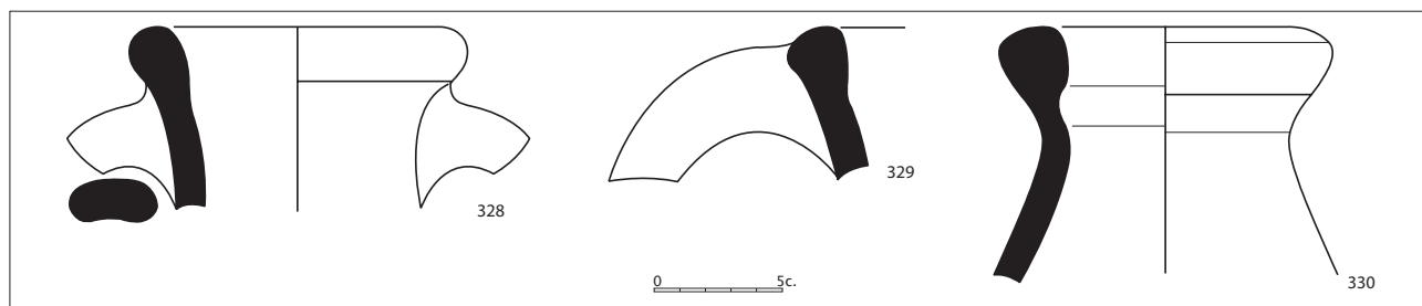
Figura 2.75. Àmfores Keay 36 B.
